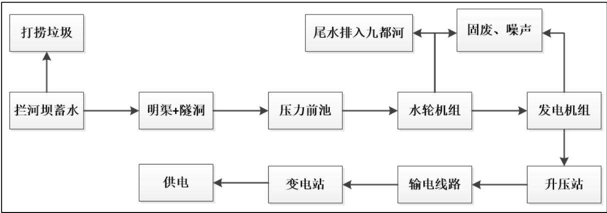
图 4.3-1 工艺流程及产污节点图
