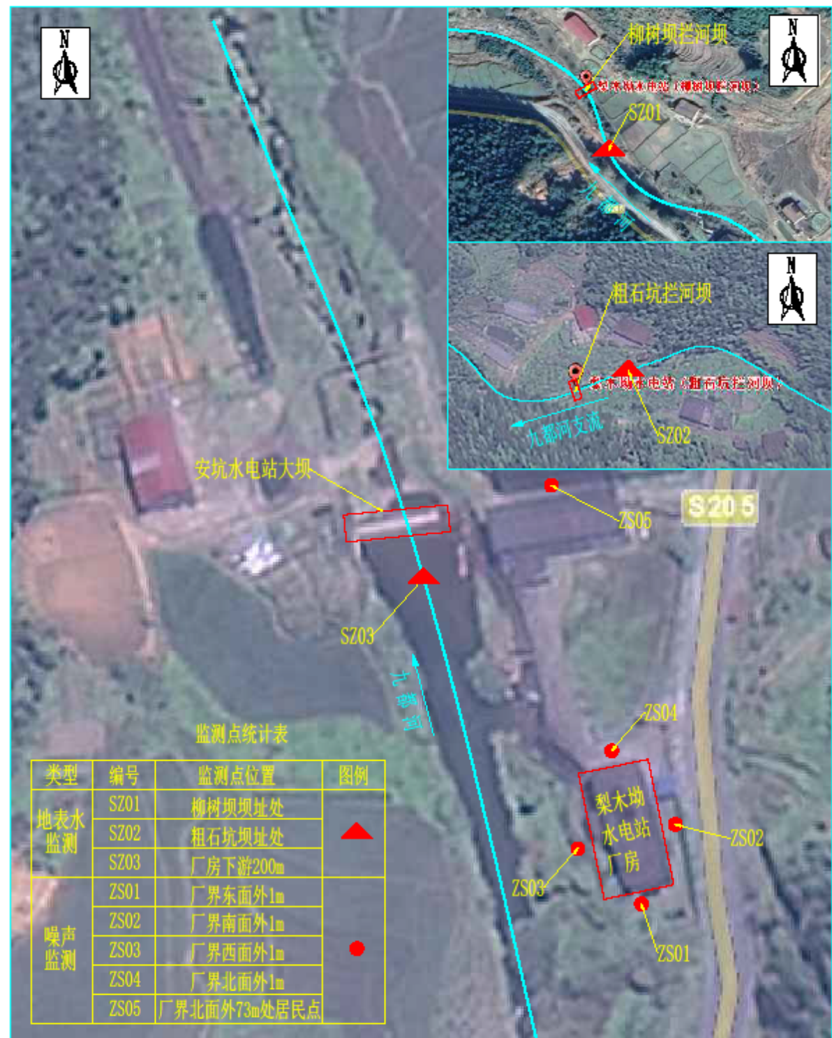
附图 5 监测点位布置图
