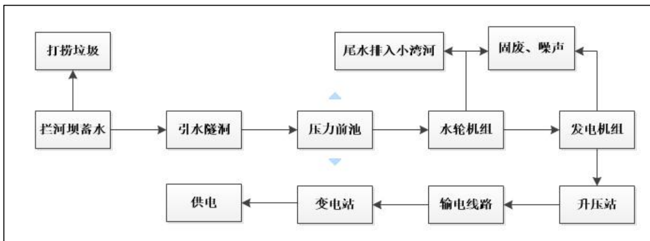
图 4.3-1 工艺流程及产污节点图
