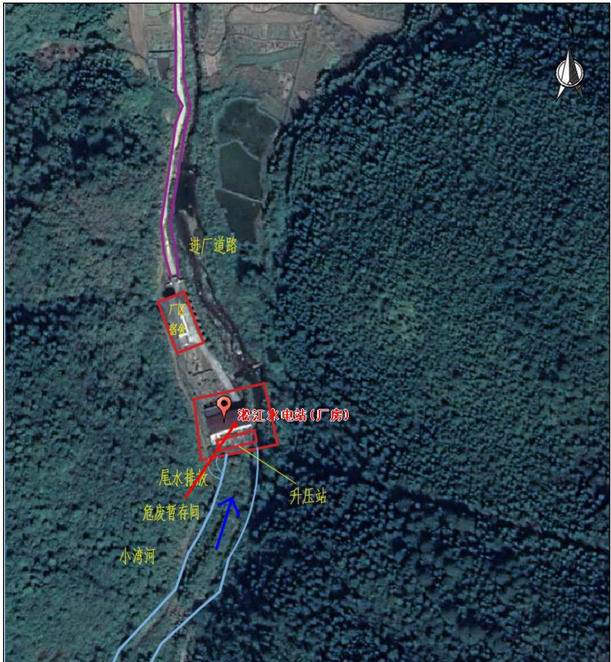
附图3 厂区平面布置图
