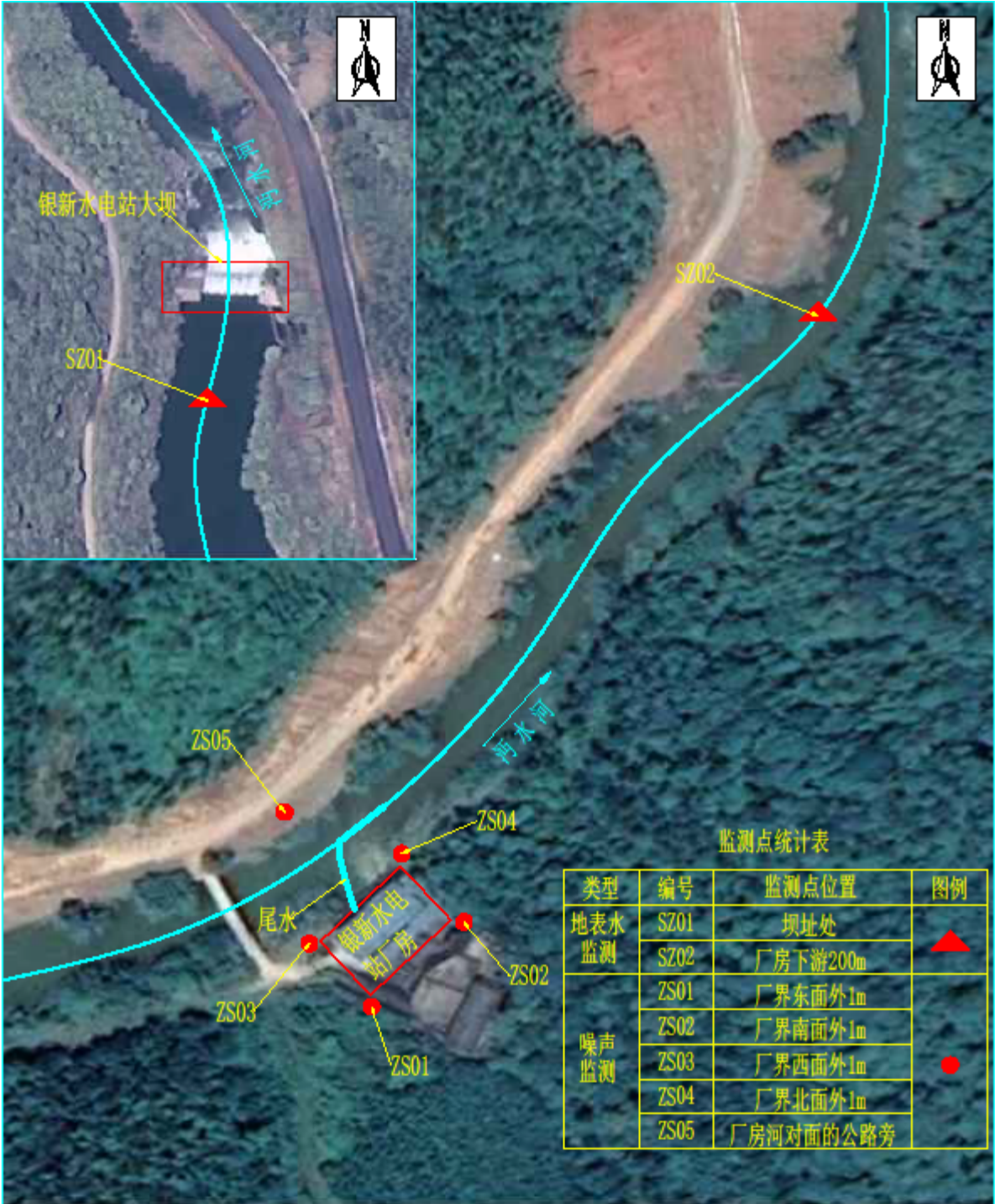
附图 5 监测点位布置图
