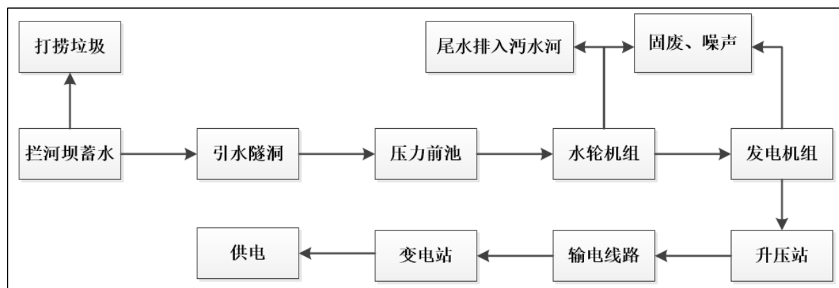
图 4.3-1 工艺流程及产污节点图
