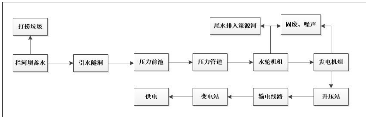
图 4.3-1 工艺流程及产污节点图
