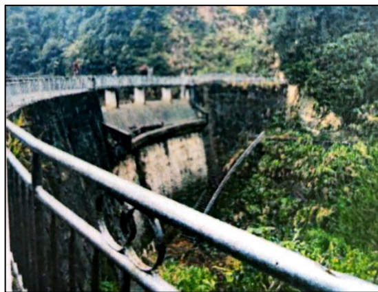
大源水电站大坑拦河坝
