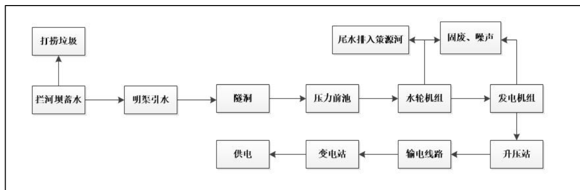
图 4.3-1 工艺流程及产污节点图
