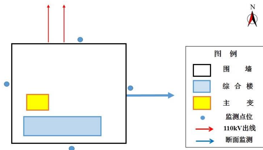
图 10 回龙 110kV 变电站平面布置及监测点位示意图
