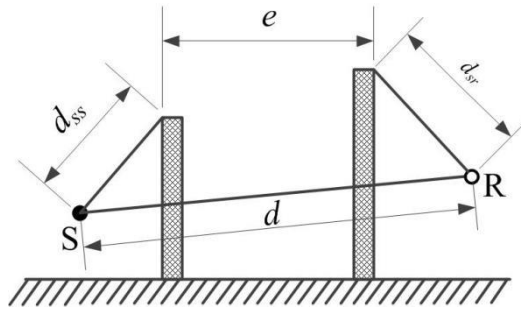
图 8 利用建筑物、土堤作为厚屏障
