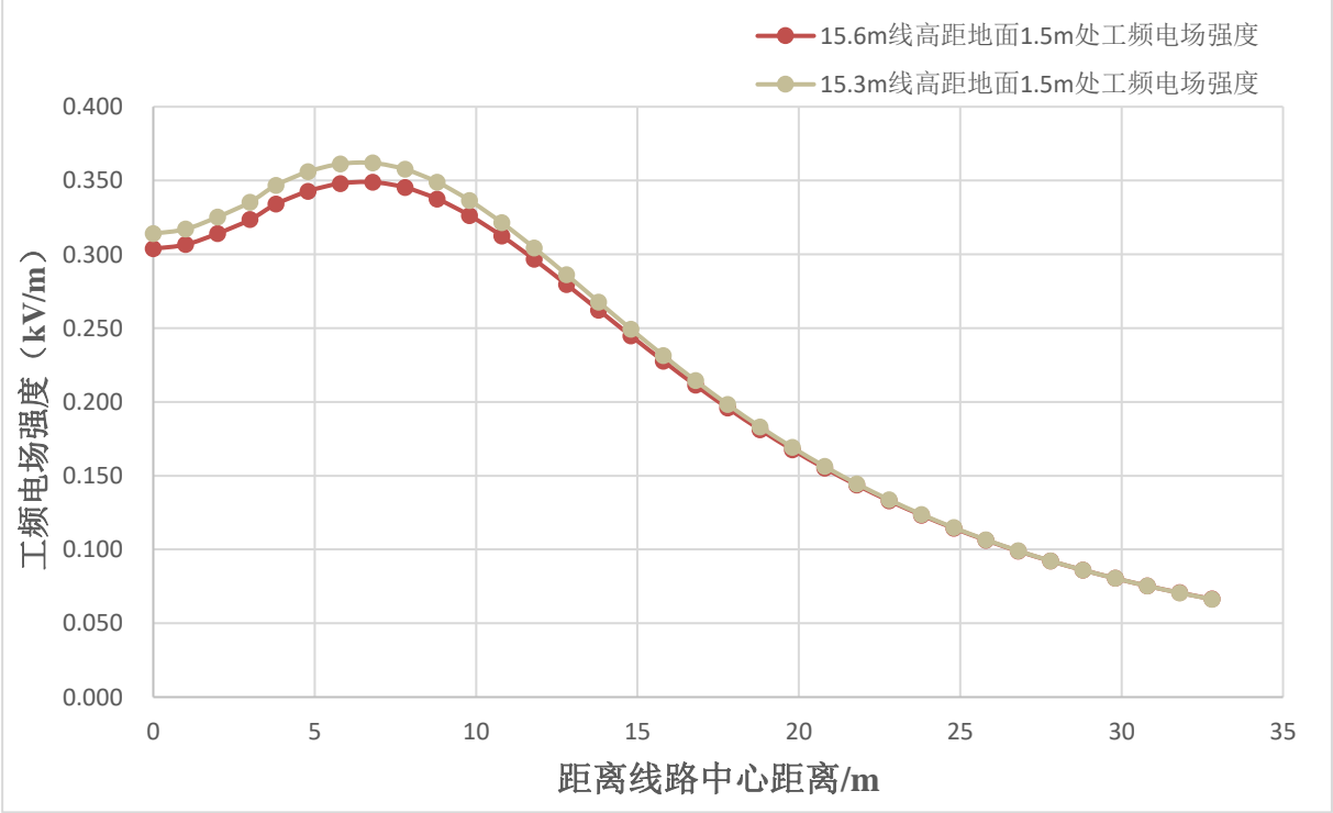
图 15 110kV 架空线路工频电场预测结果
