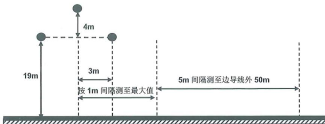
图 11 110kV 沈宝新线电磁衰减断面监测示意图
