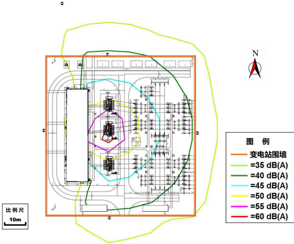
图 9 新市 110kV 变电站本期规模噪声预测等值线图
