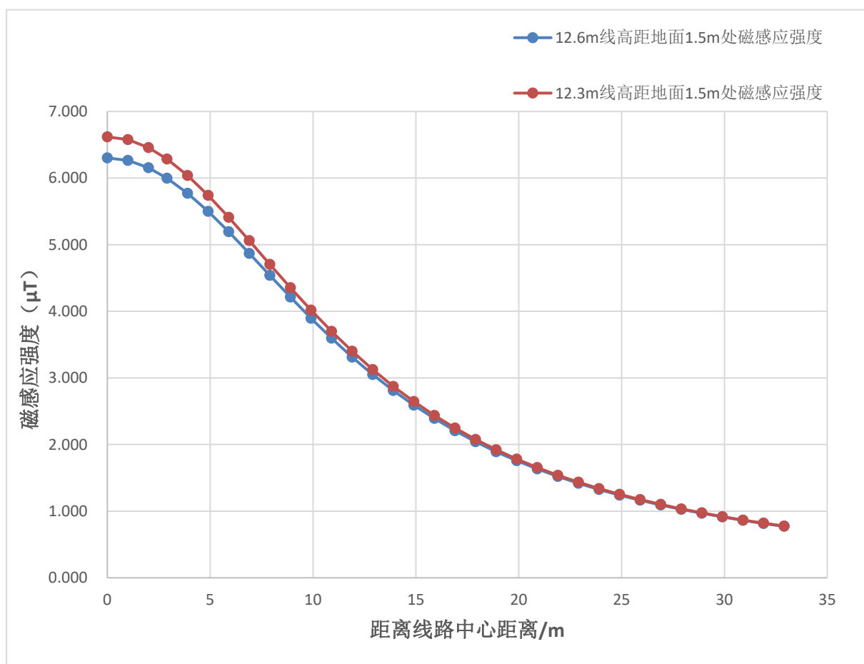
图 14 110kV 架空线路工频磁场预测结果
