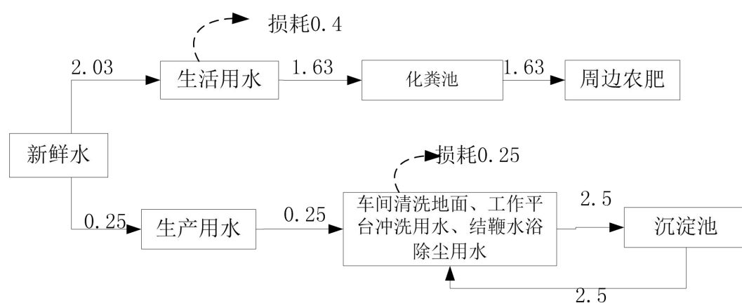
图 2-1a 变更后主厂区水平衡图（单位：m 3 /d）
