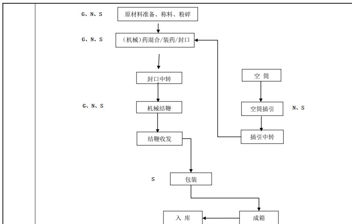
图 2-3 爆竹类 C 级产品生产工艺流程图及产污节点图 工艺流程简述
