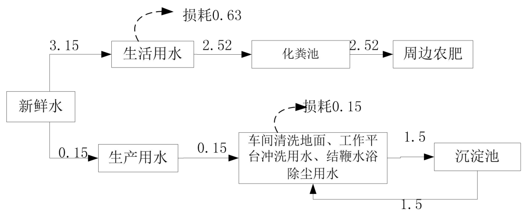
图 2-1b 变更后斋江工区水平衡图（单位：m 3 /d）
