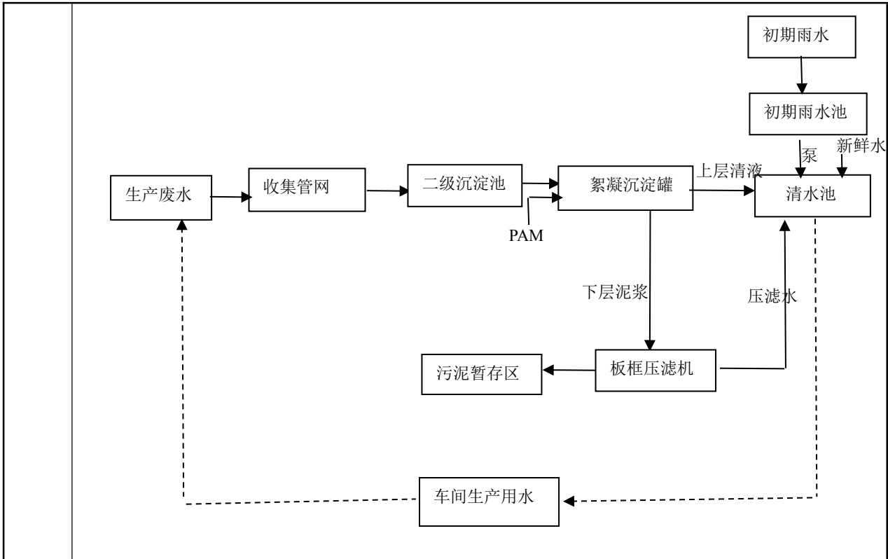
图 4-3 项目废水处理及回用工艺流程示意图
