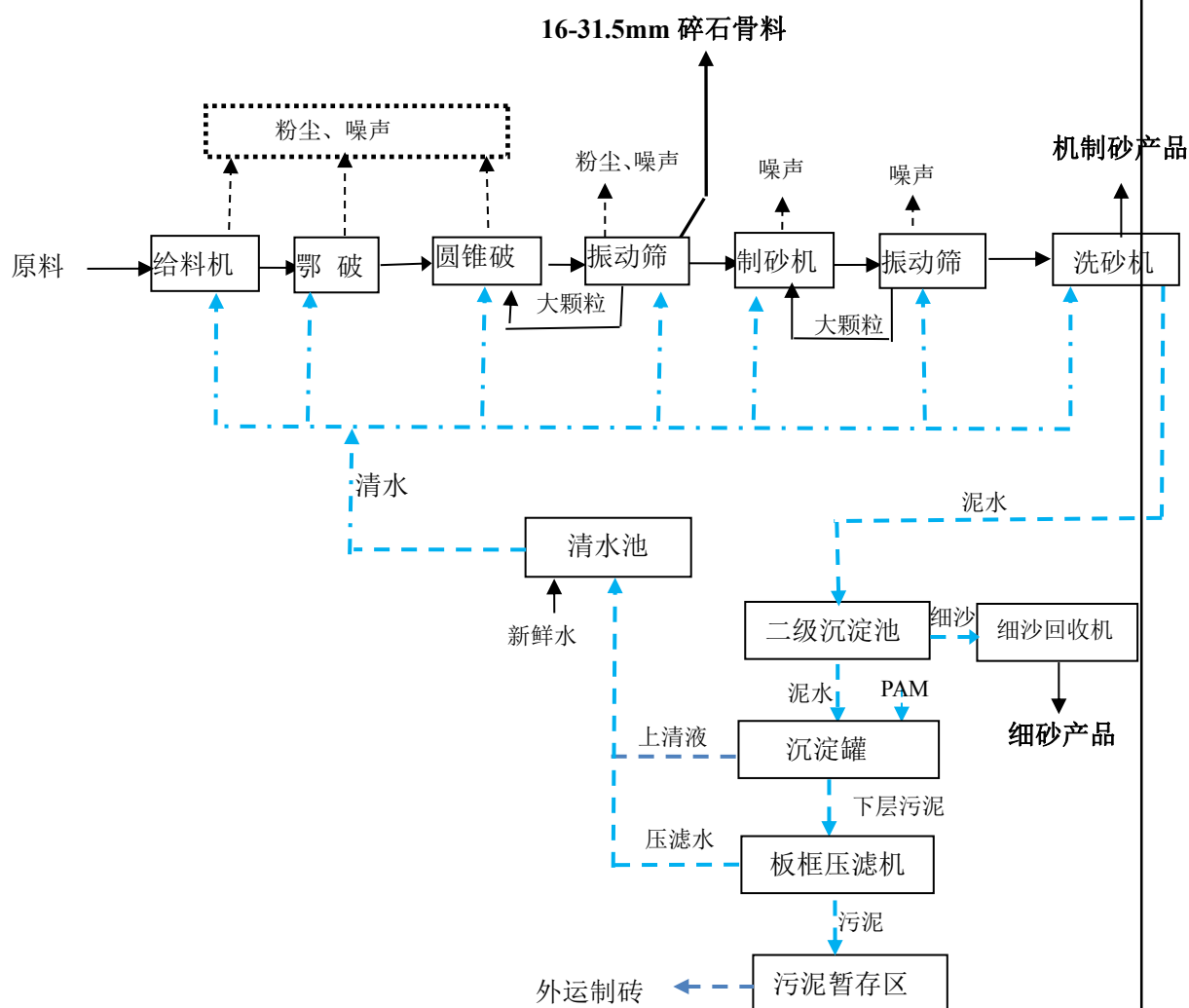
图 2-2 营运期工艺流程及产污环节节点示意图
