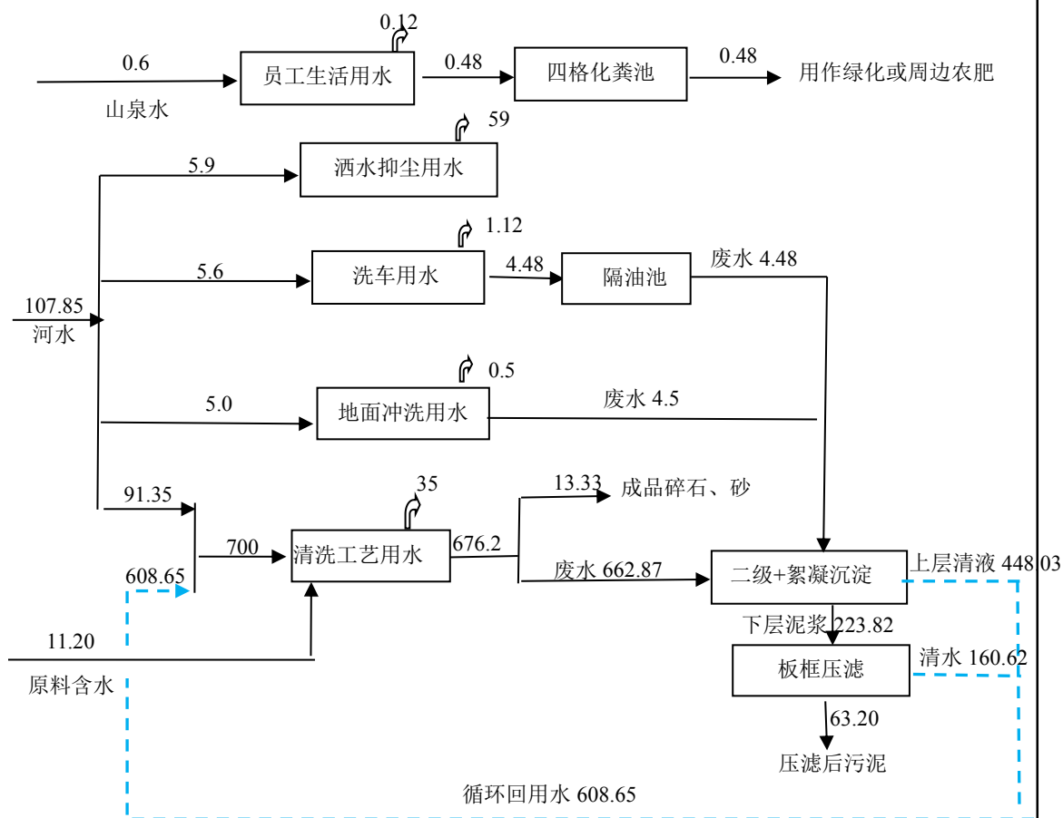
图 4-1 项目用排水平衡图（未含初期雨水） 单位 m 3 /d
