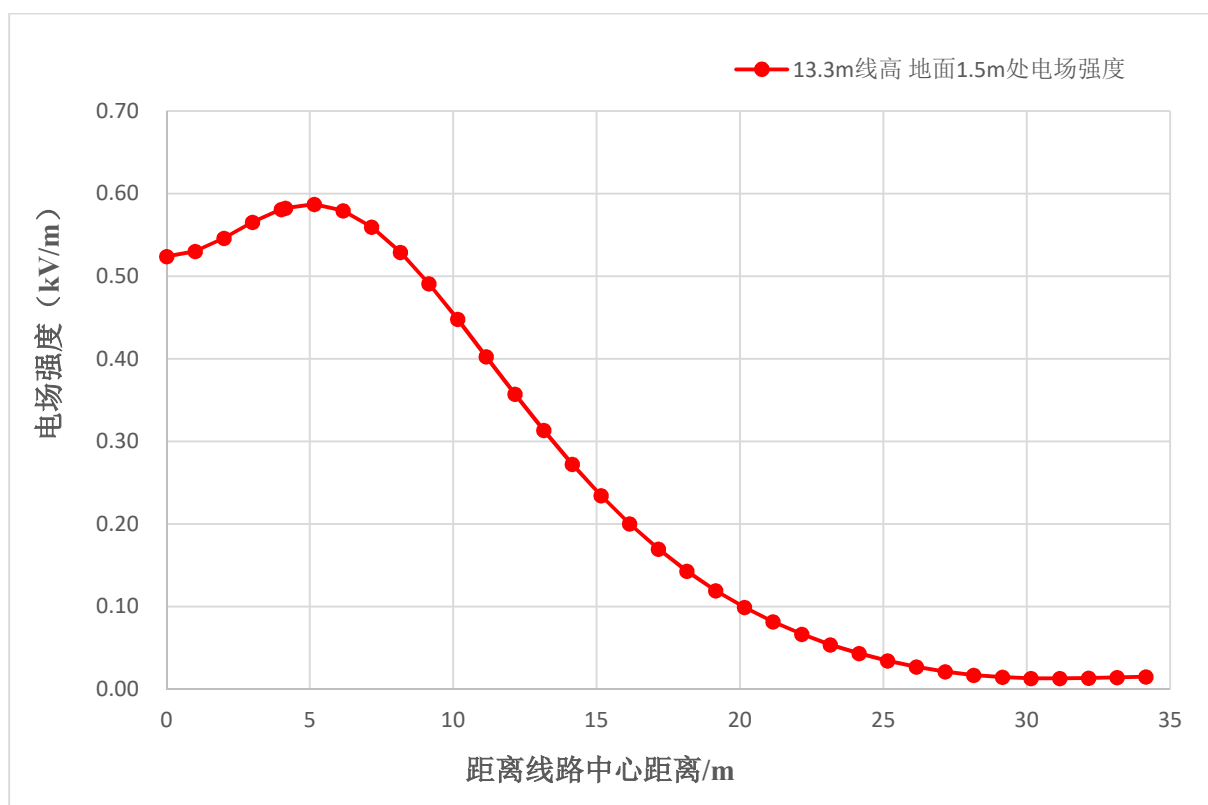
图 13 110kV 同塔双回线路电场强度预测结果
