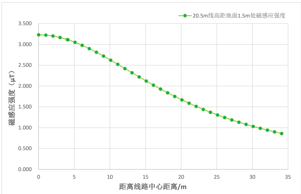
图 16 110kV 单回线路磁感应强度预测结果
