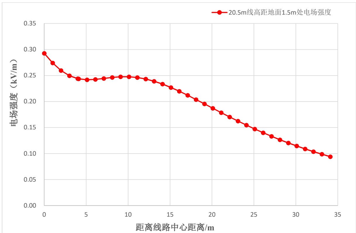
图 15 110kV 单回线路电场强度预测结果
