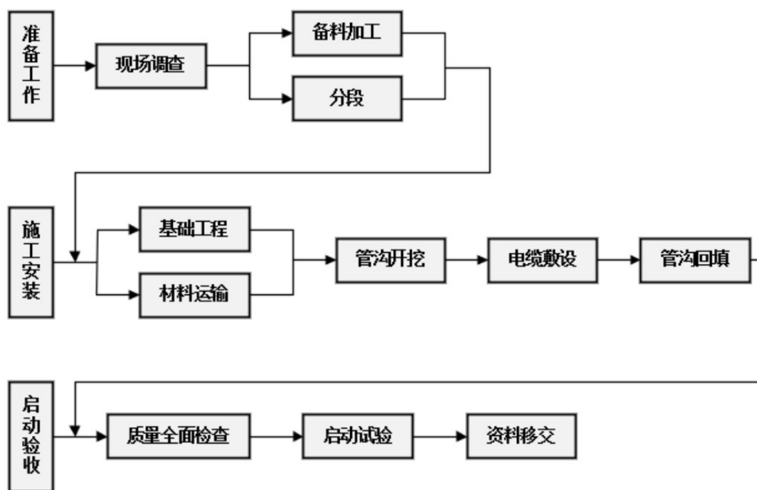
图 3 电缆线路施工工艺流程
