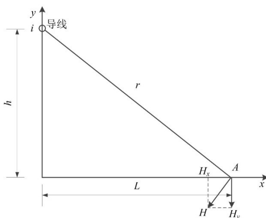
图 12 磁场向量图
