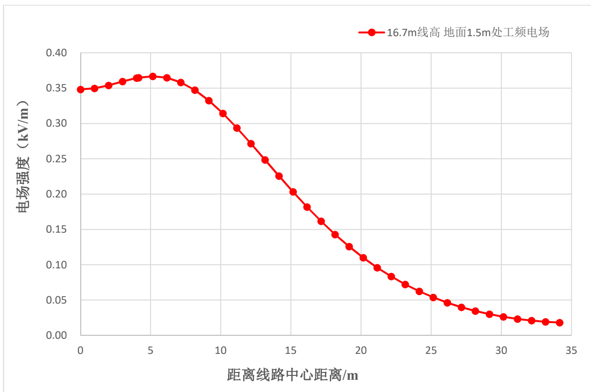
图 17 110kV 同塔双回线路电场强度预测结果
