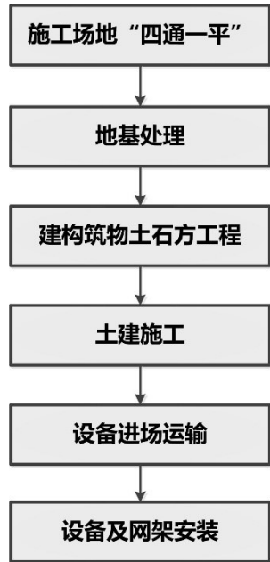
图 1 变电站工程施工工艺流程
