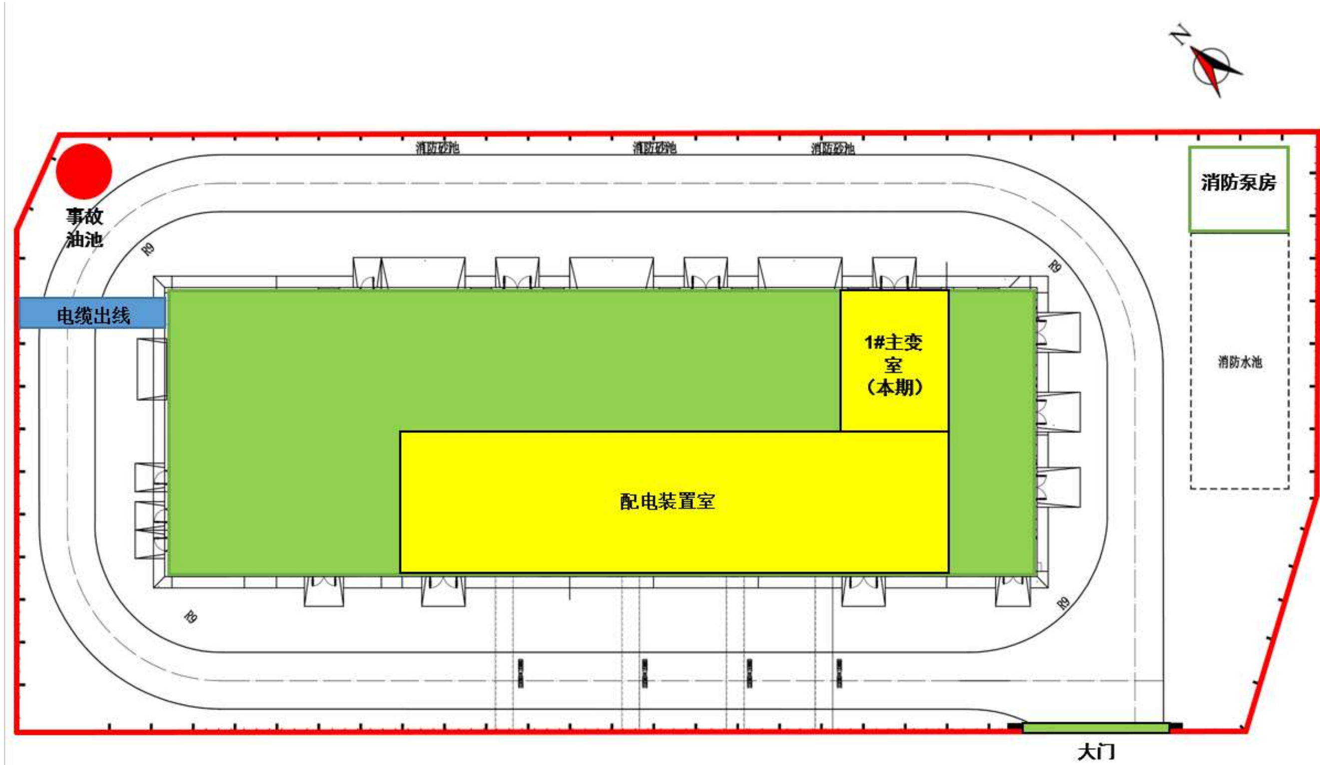
附图 2：金山 110kV 变电站总平面布置示意图
