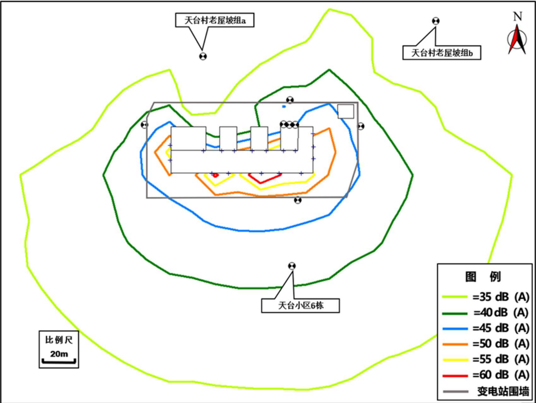
图 10 金山 110kV 变电站噪声预测等值线图
