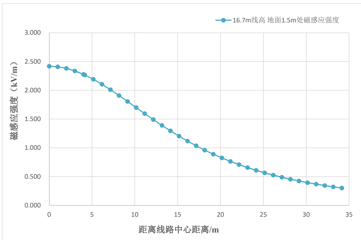
图 18 110kV 同塔双回线路磁感应强度预测结果
