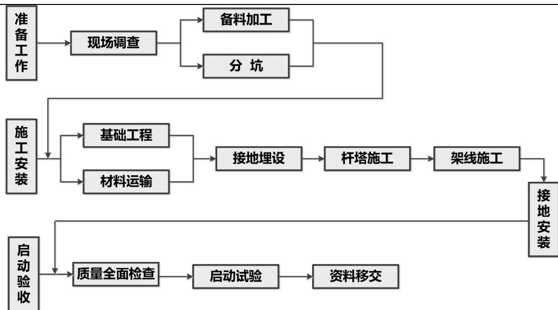
图 2 架空线路施工工艺流程
