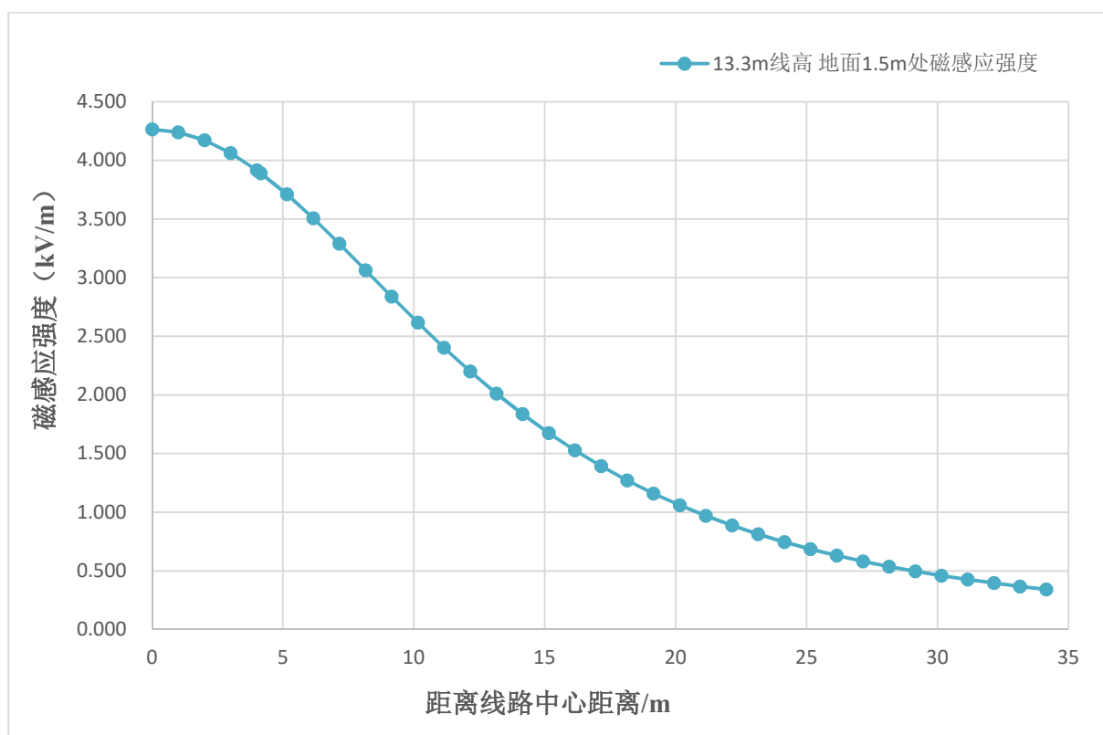
图 14 110kV 同塔双回线路磁感应强度预测结果
