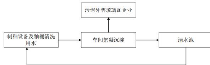
图2.1-4 制釉废水处理工艺流程图
