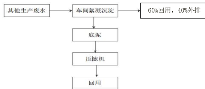
图2.1-5 污水处理站处理工艺流程图
