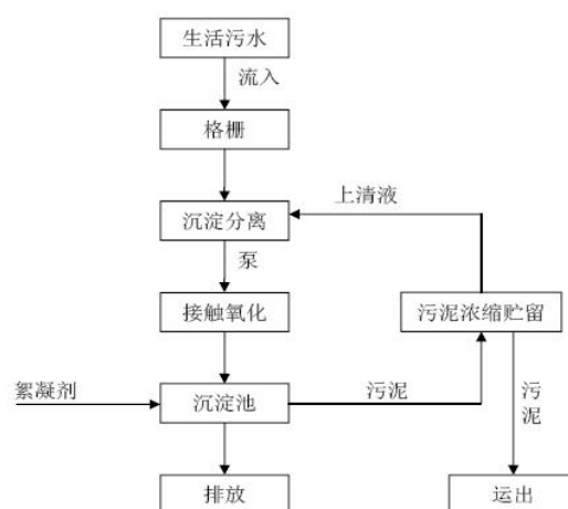
图2.1-3 生活污水处理工艺流程图
