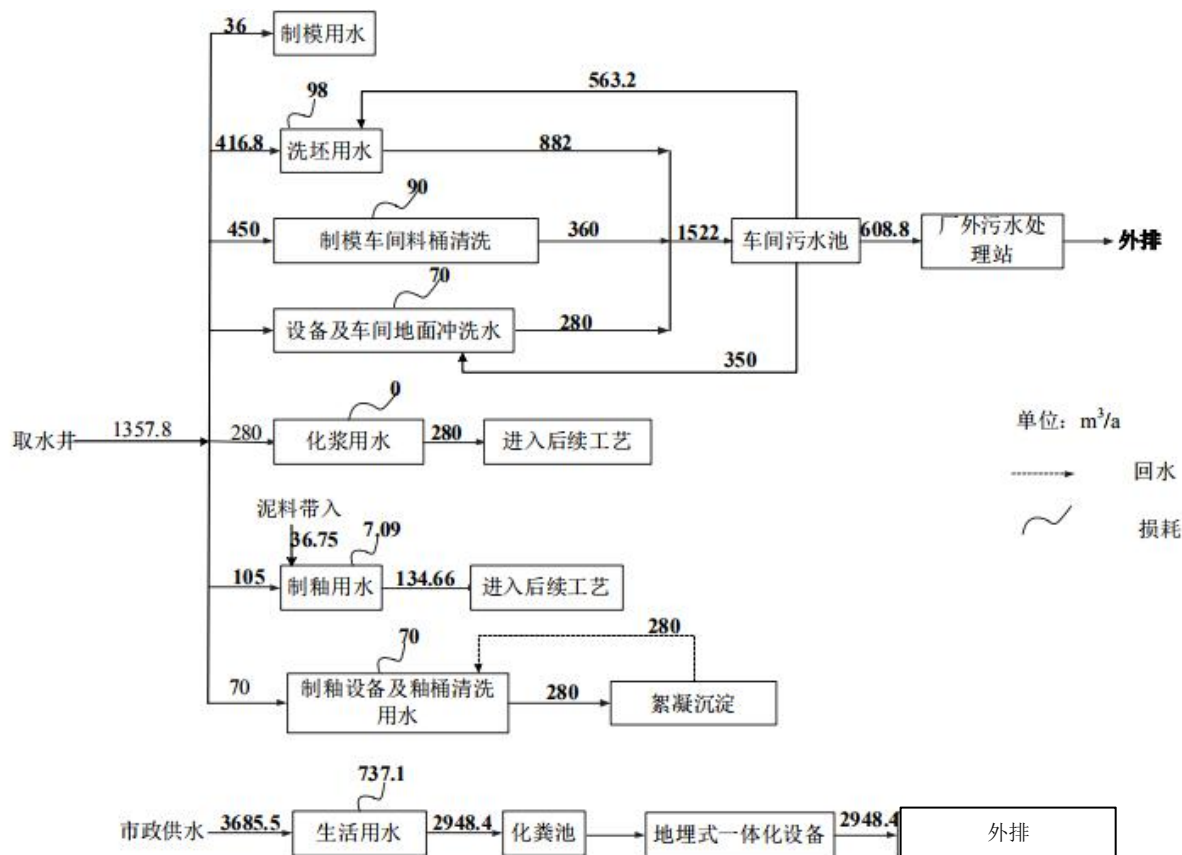
图2.1-2 项目水平衡图
