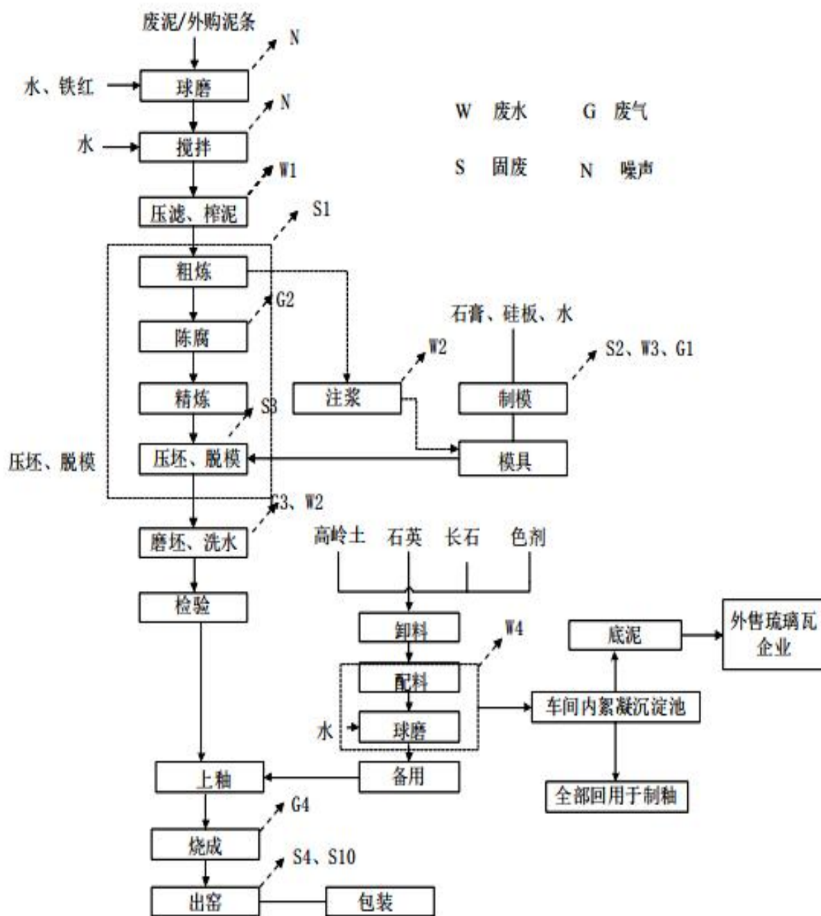
图2.1-1 生产工艺流程及产污节点图
