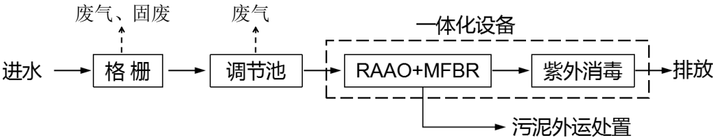
图 2-3 处理规模为 500m 3 /d 及以下乡镇污水处理厂工艺流程简图
