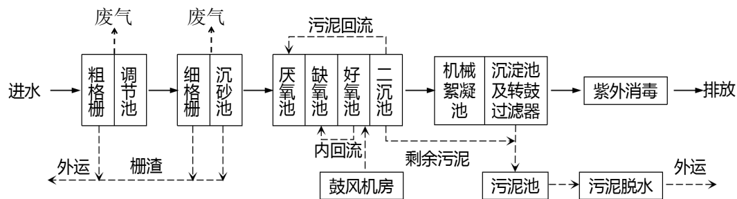
图 2-4 处理规模为 500m 3 /d 以上乡镇污水处理厂工艺流程简图
