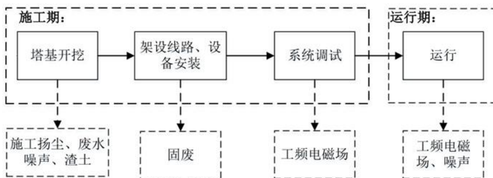
图 1 项目建设流程和产污节点图
