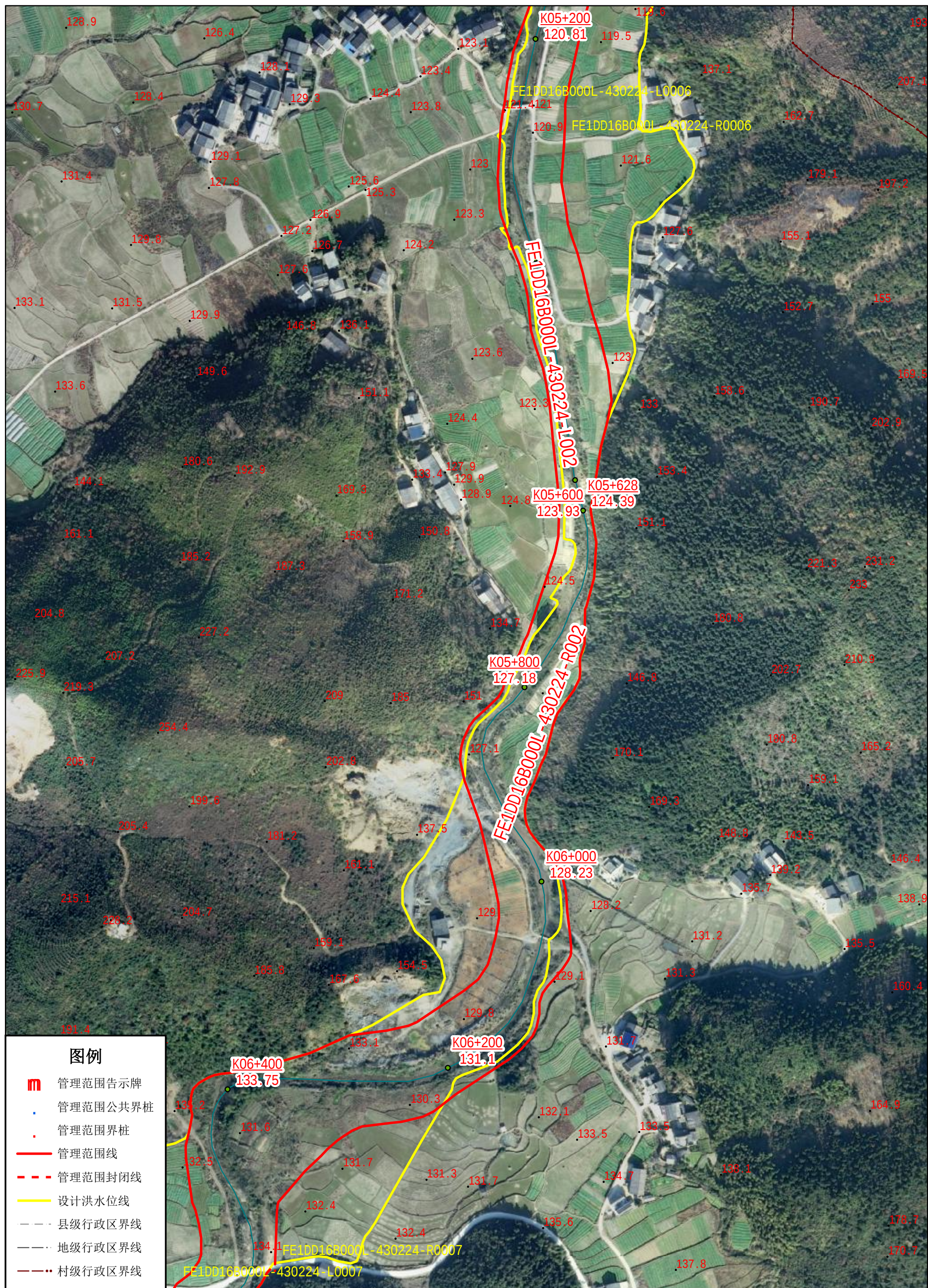
茶陵县把集江河道管理范围划定图(五)
