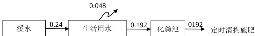
图 2.6-1 项目水平衡图（m 3 /d）
