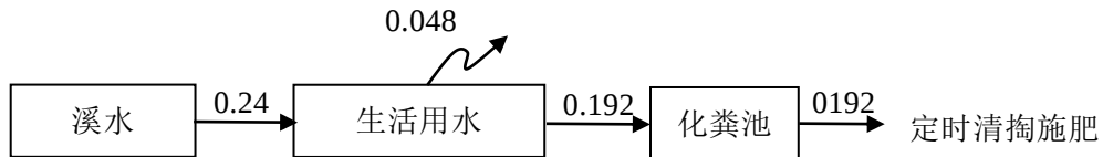
图 2.6-1 项目水平衡图 ( \text{m}^3/\text{d} )
