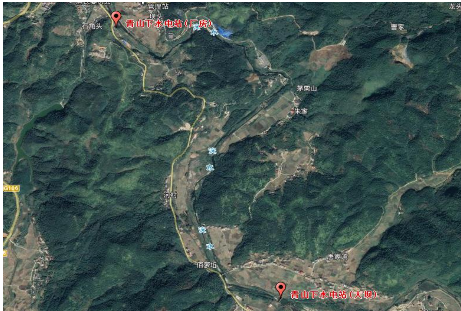
图 3.2.1 电站大坝及厂址位置示意图
