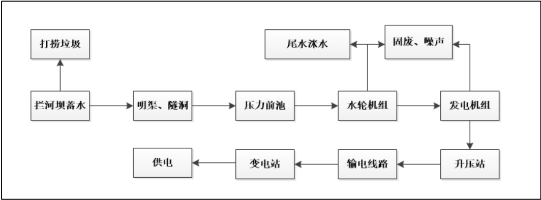
图 4.3-1 工艺流程及产污节点图
