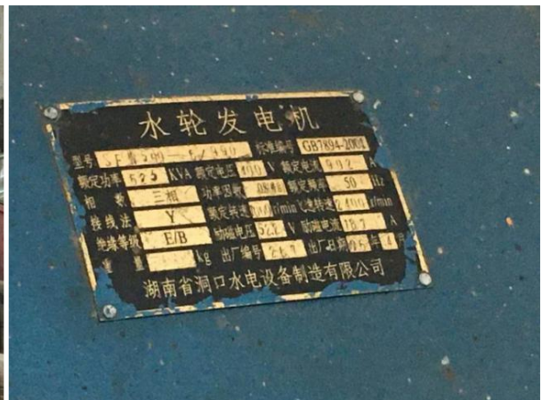
厂房内水轮机铭牌
