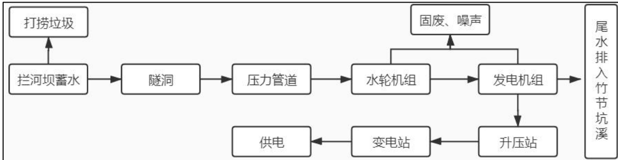
图 4.3-1 工艺流程及产污节点图
