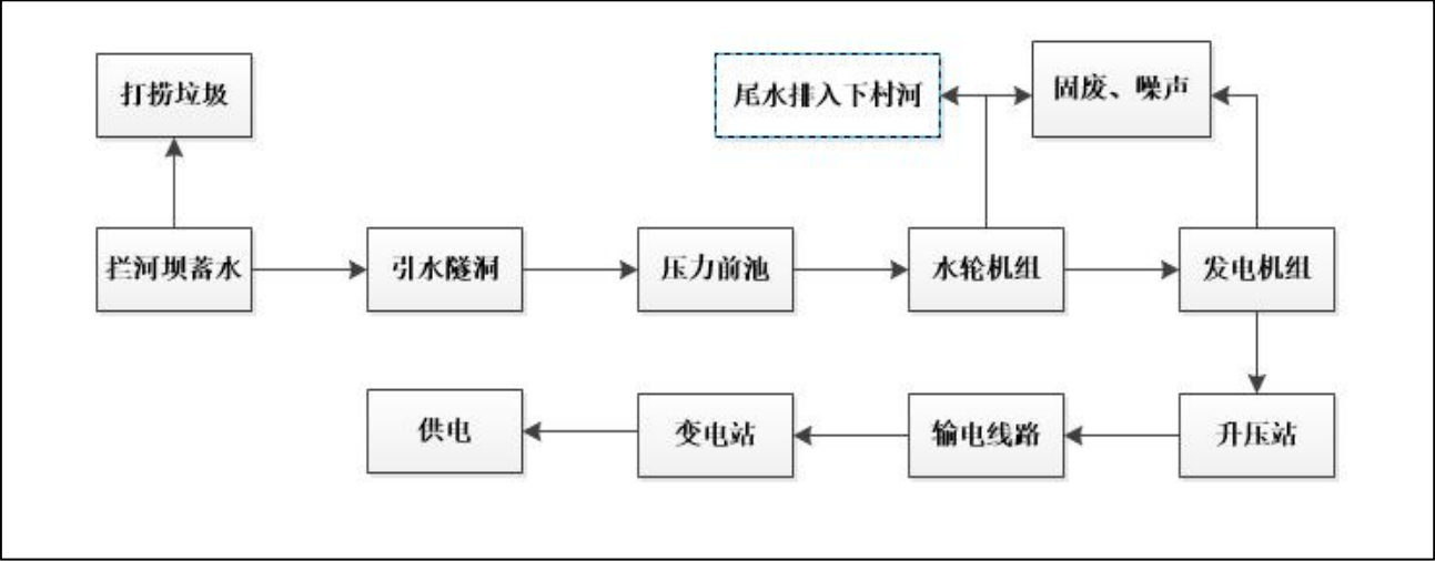
图 4.3-1 工艺流程及产污节点图
