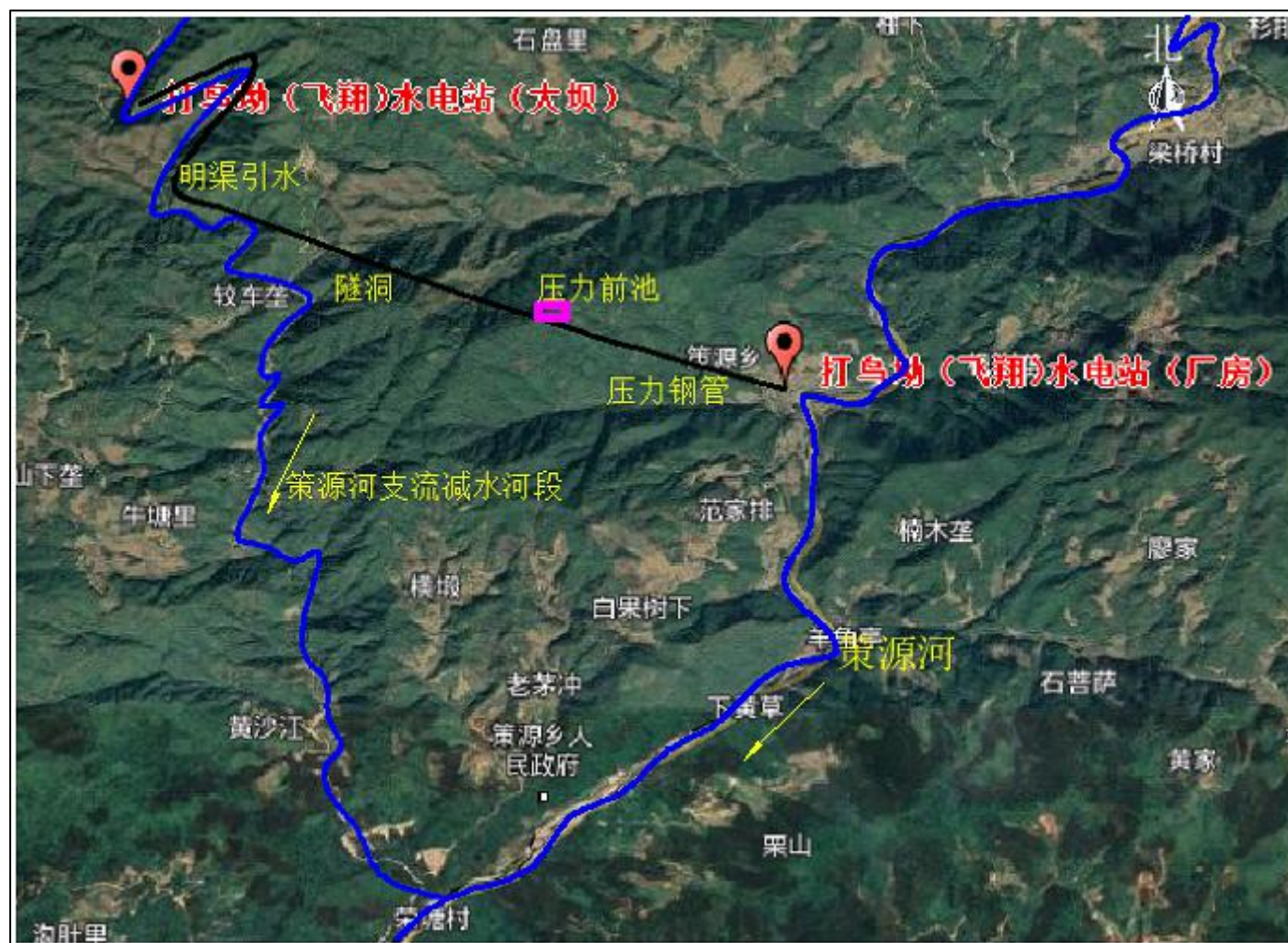
附图 3 工程总体平面布置图
