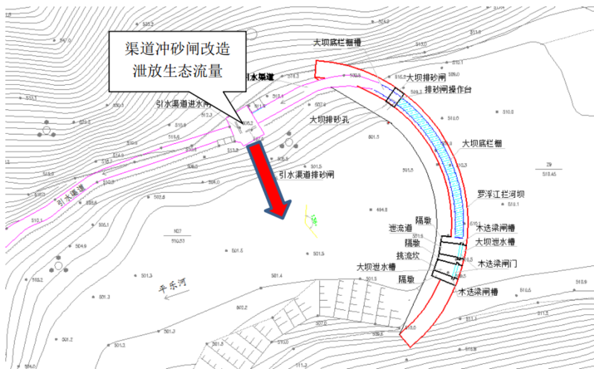
图 5.1-1 渠道冲砂闸改造方案示意图
