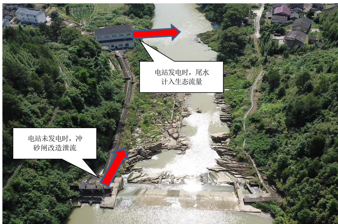
图 5.1-1 生态基荷+冲砂闸改造联动方案示意图
