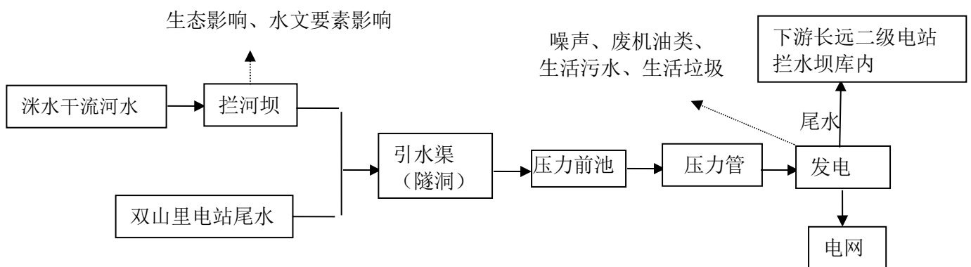
图3.2-1 电站工艺流程及产污节点示意图
