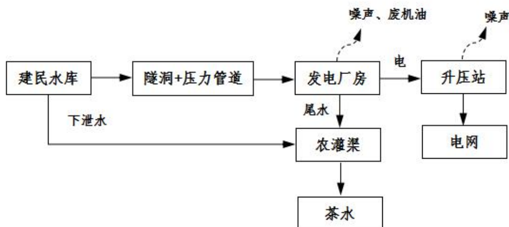
图 5-1. 工艺流程及产污环节图
