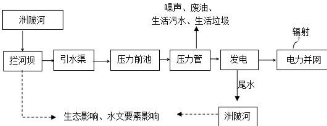
图 5-1. 工艺流程及产污环节图
