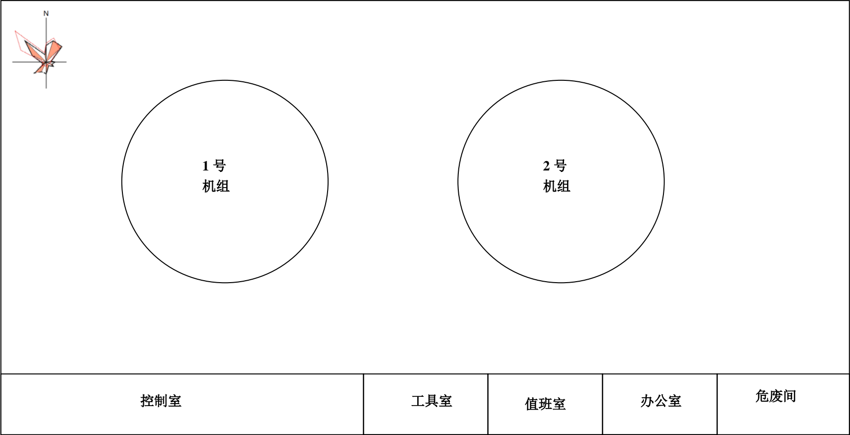
附图4. 厂房平面布置图
