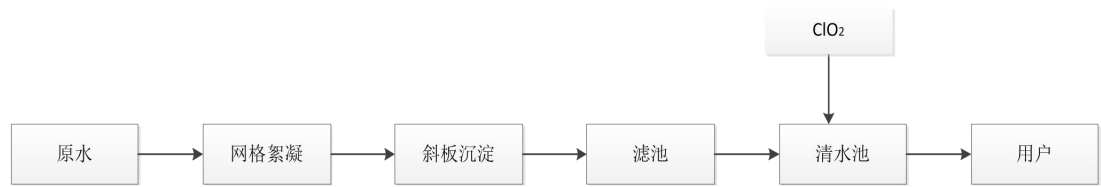
图 2-1 水厂工艺流程示意图
