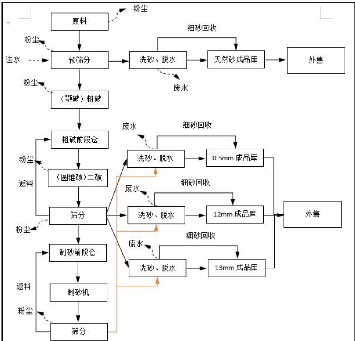
图 5-2 一期工程生产工艺流程图
