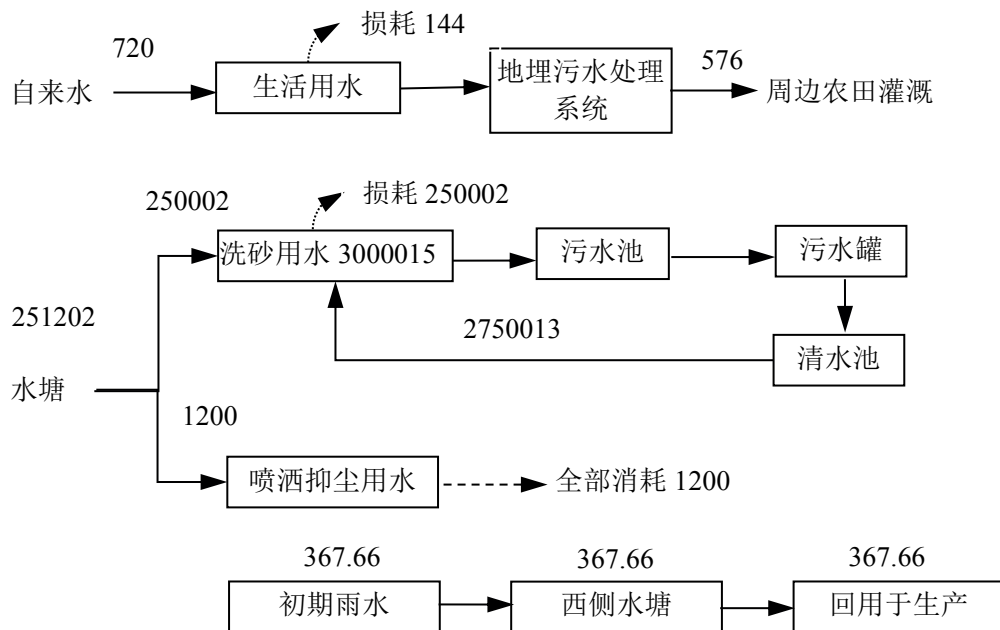
图 1-1 项目水平衡图（晴天）单位 t/a
