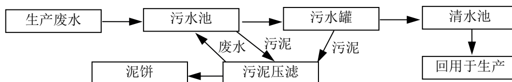
图 7-1 项目生产污水处理工艺流程图
