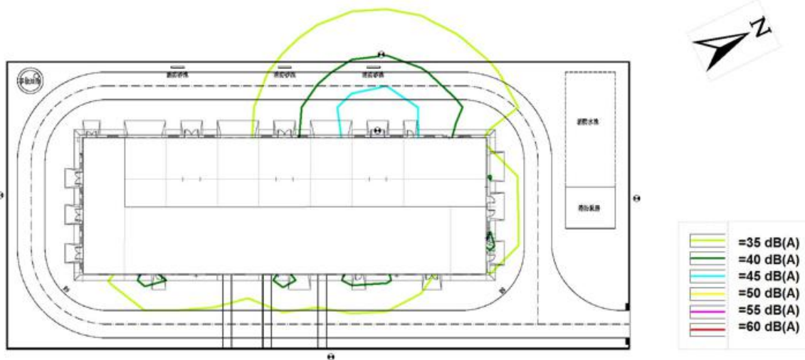
图 8 托福 110kV 变电站本期规模噪声预测等值线图
