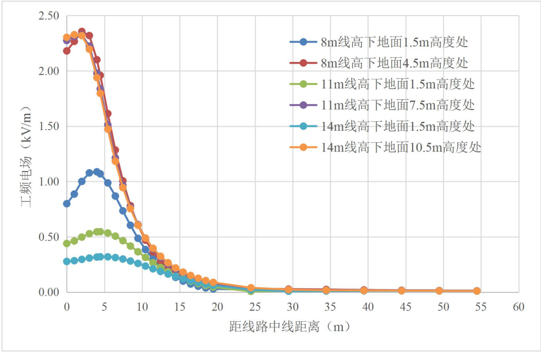
图 15 110kV 同塔双回线路（典型杆塔）工频电场预测分布图
