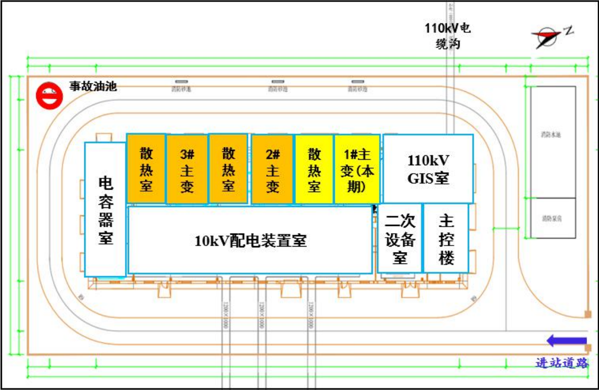
图 2 托福 110kV 变电站总平面布置示意
