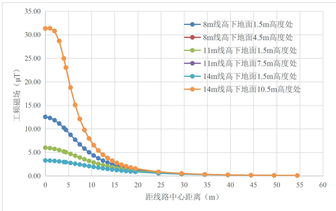
图 16 110kV 同塔双回线路（典型杆塔）工频磁场预测分布图
