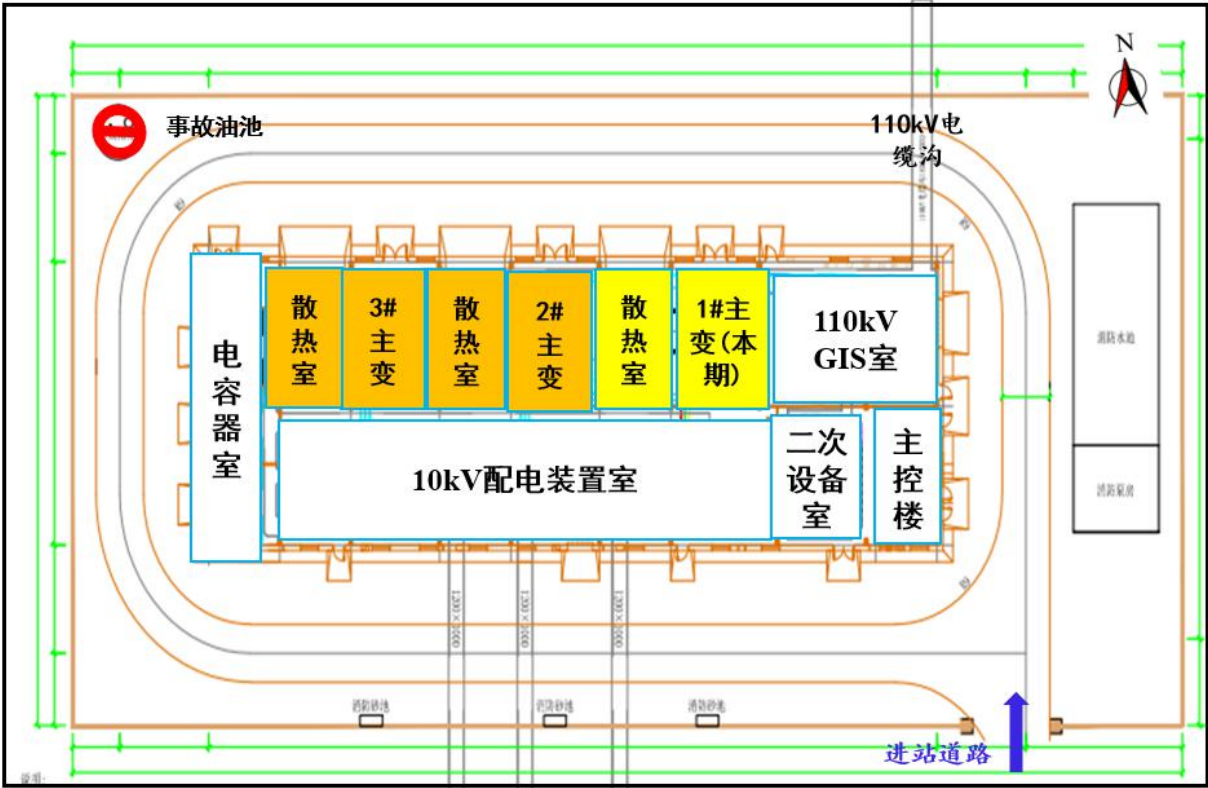
图 2 黄沙 110kV 变电站总平面布置示意
