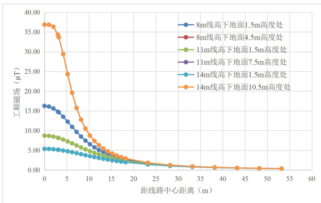
图 16 110kV 单回线路（典型杆塔）工频磁场预测分布图
