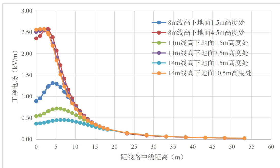
图 15 110kV 单回线路（典型杆塔）工频电场预测分布图
