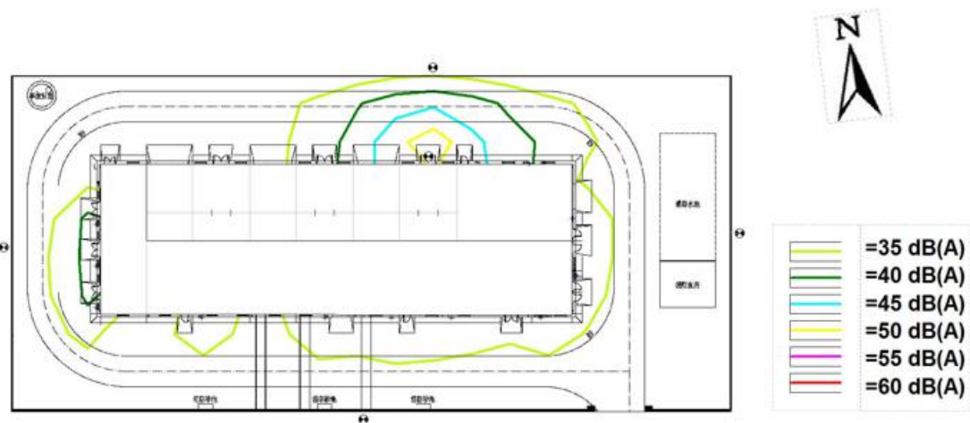
图 8 黄沙 110kV 变电站本期规模噪声预测等值线图
