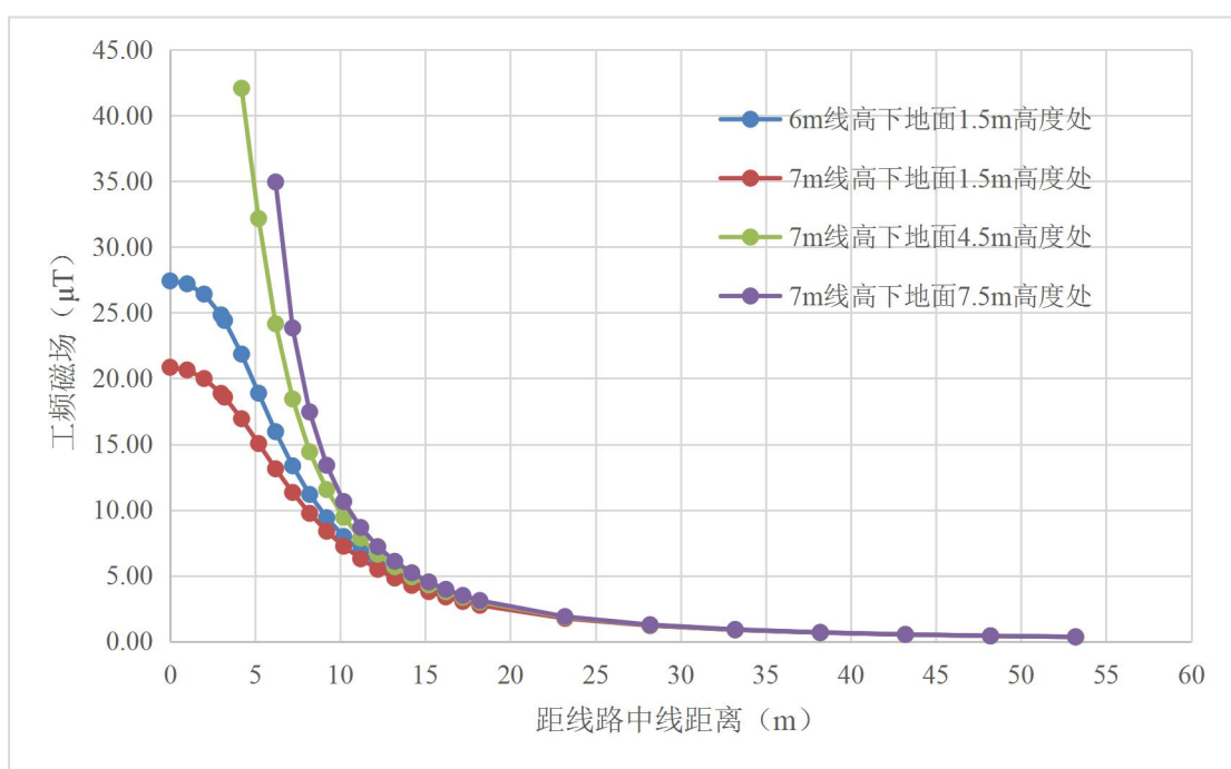
图 14 110kV 单回线路（典型杆塔）磁感应强度预测分布图
