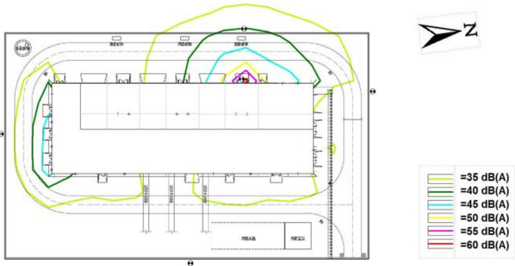
图 8 高福 110kV 变电站本期规模噪声预测等值线图
