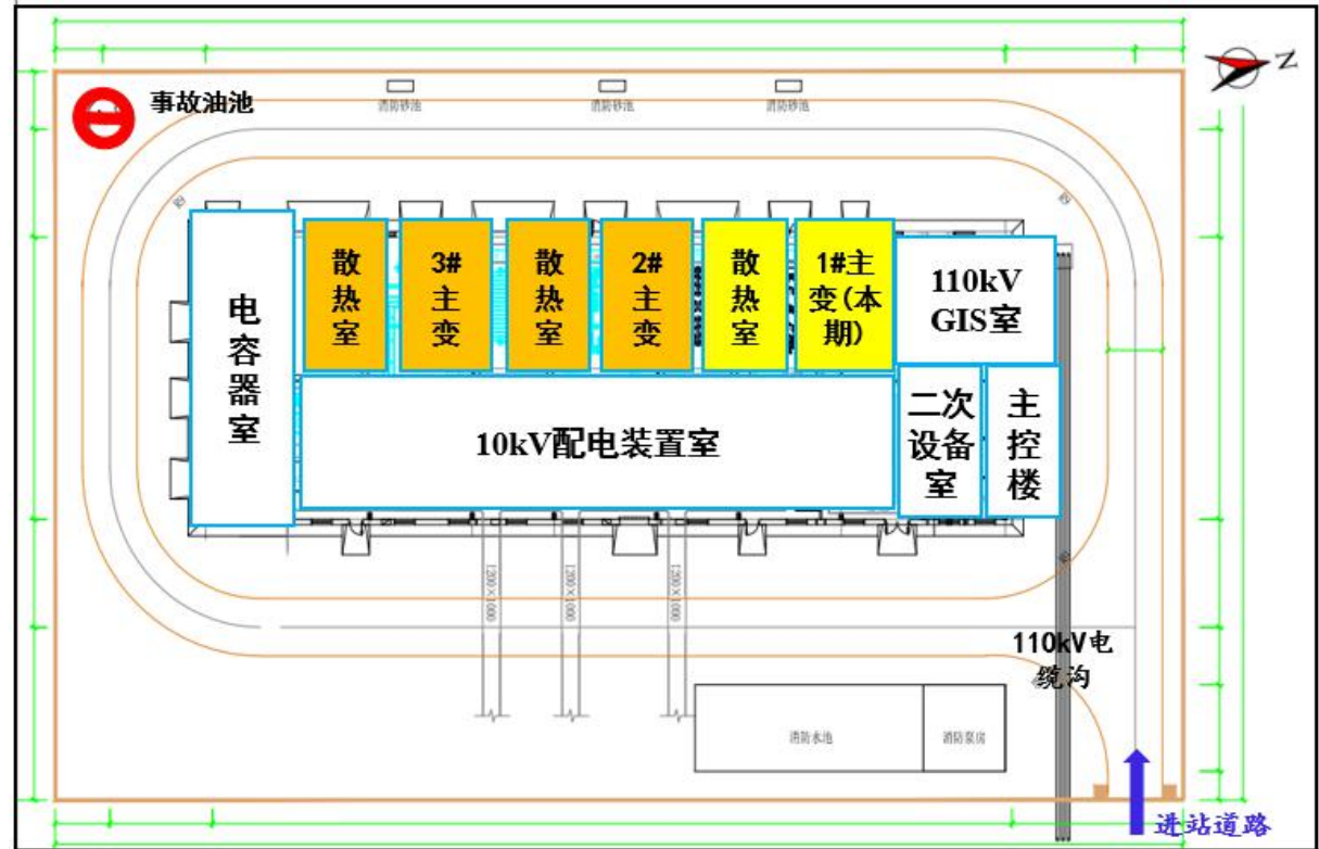
图 2 高福 110kV 变电站总平面布置示意
