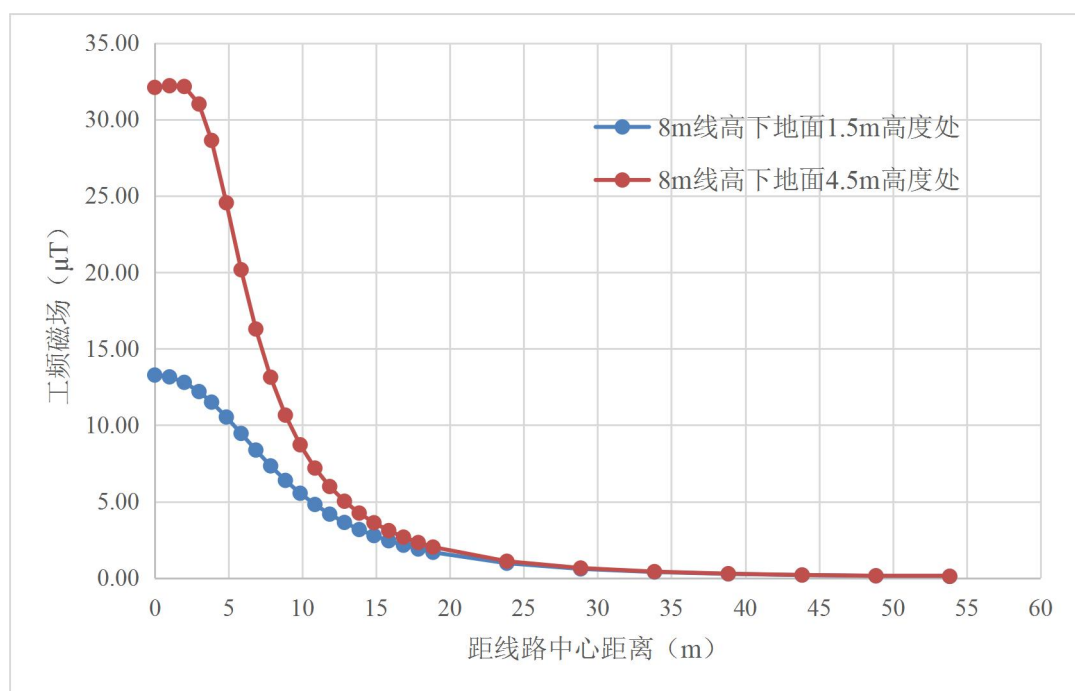
图 16 110kV 双回线路（典型杆塔）工频磁场预测分布图
