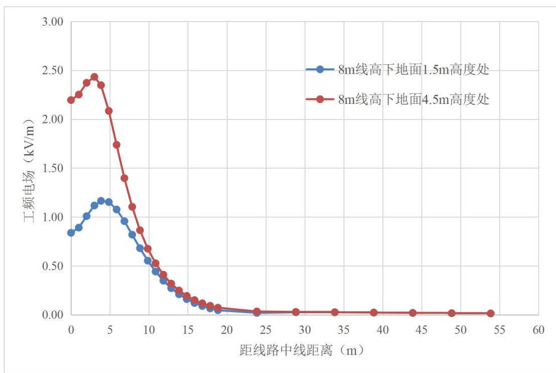
图 15 110kV 双回线路（典型杆塔）工频电场预测分布图
