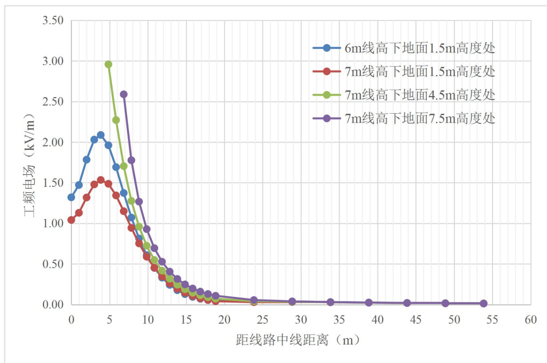
图 13 110kV 同塔双回线路（典型杆塔）工频电场预测分布图
