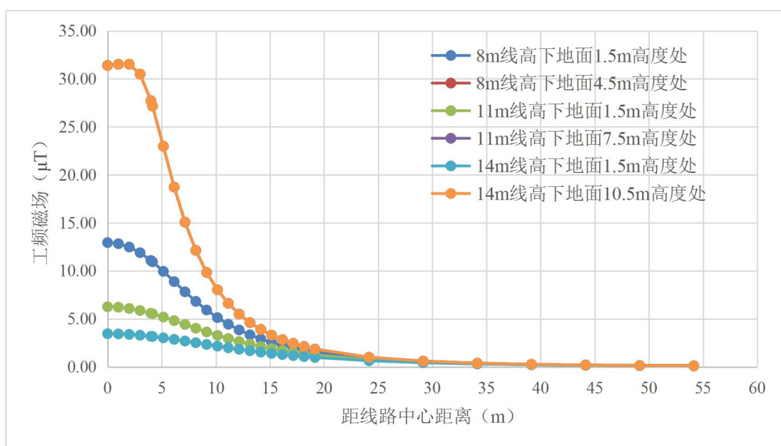
图 16 110kV 同塔双回线路（典型杆塔）工频磁场预测分布图
