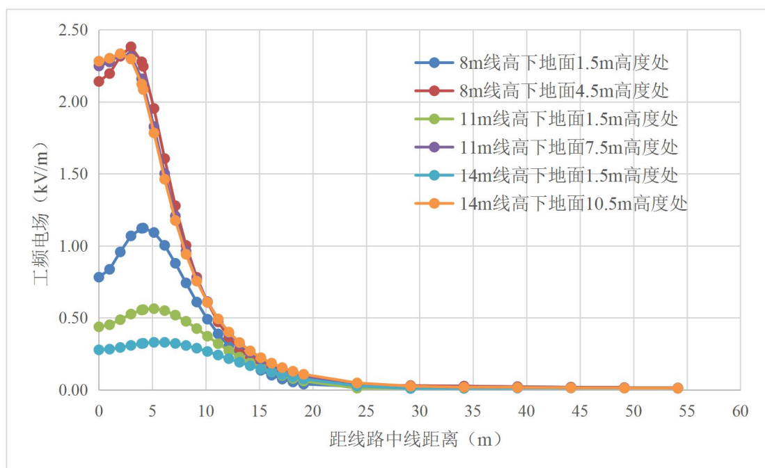
图 15 110kV 同塔双回线路（典型杆塔）工频电场预测分布图
