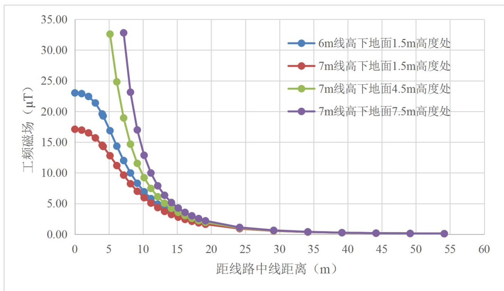
图 14 110kV 同塔双回线路（典型杆塔）磁感应强度预测分布图
