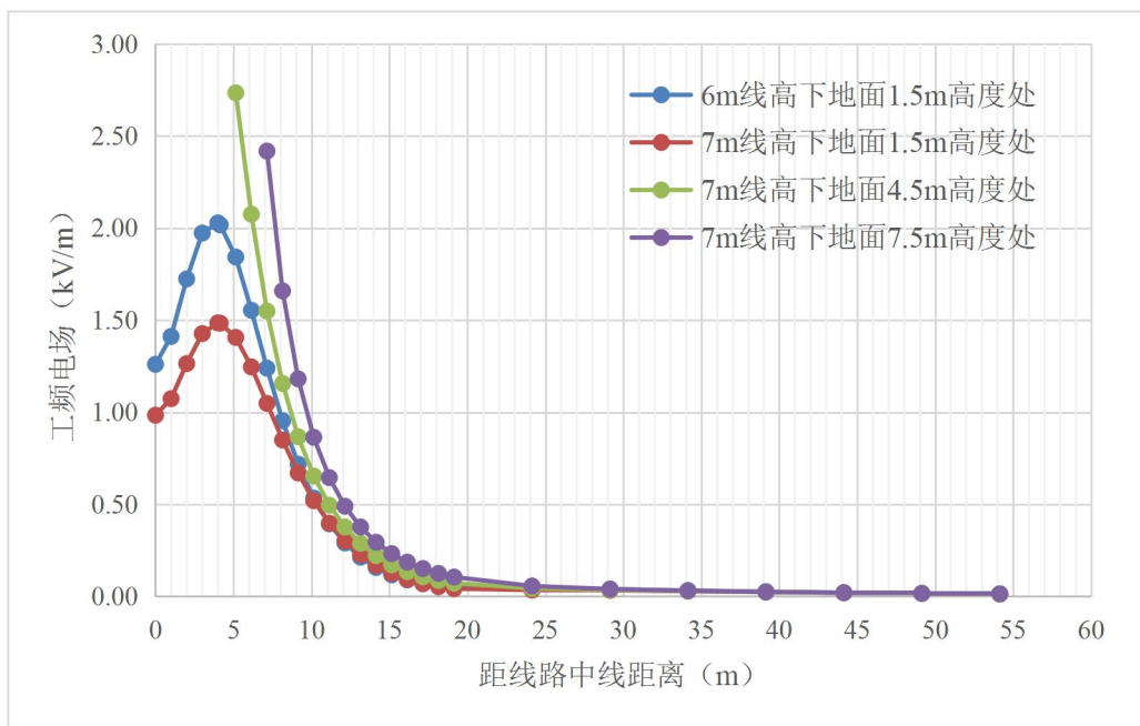
图 13 110kV 同塔双回线路（典型杆塔）工频电场预测分布图
