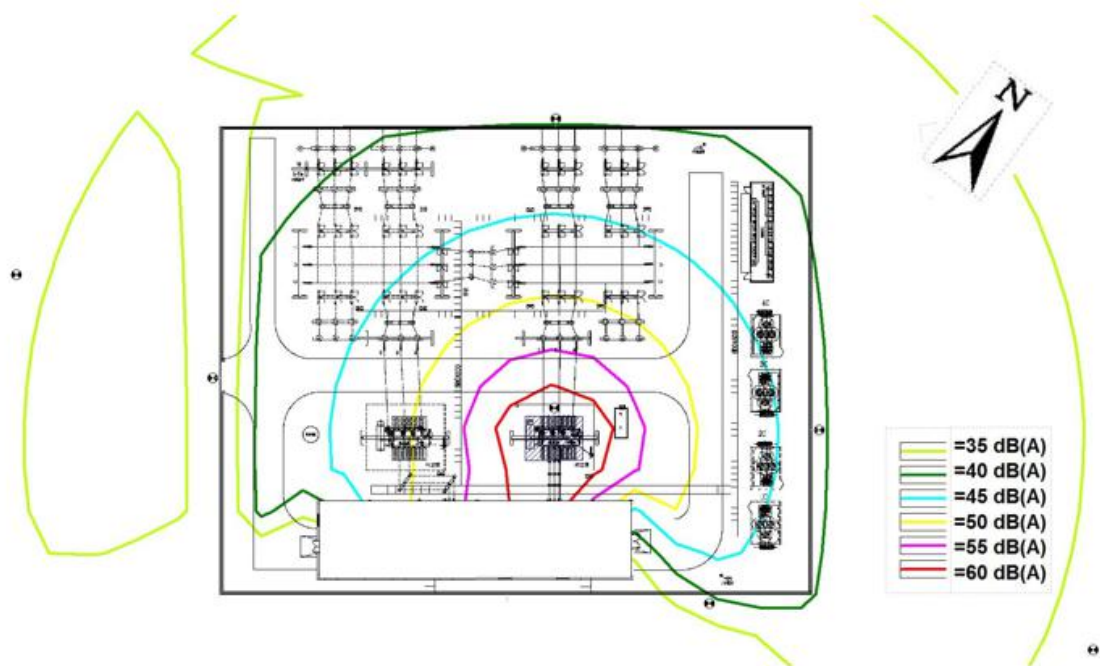
图 8 古家岭 110kV 变电站本期规模噪声预测等值线图
