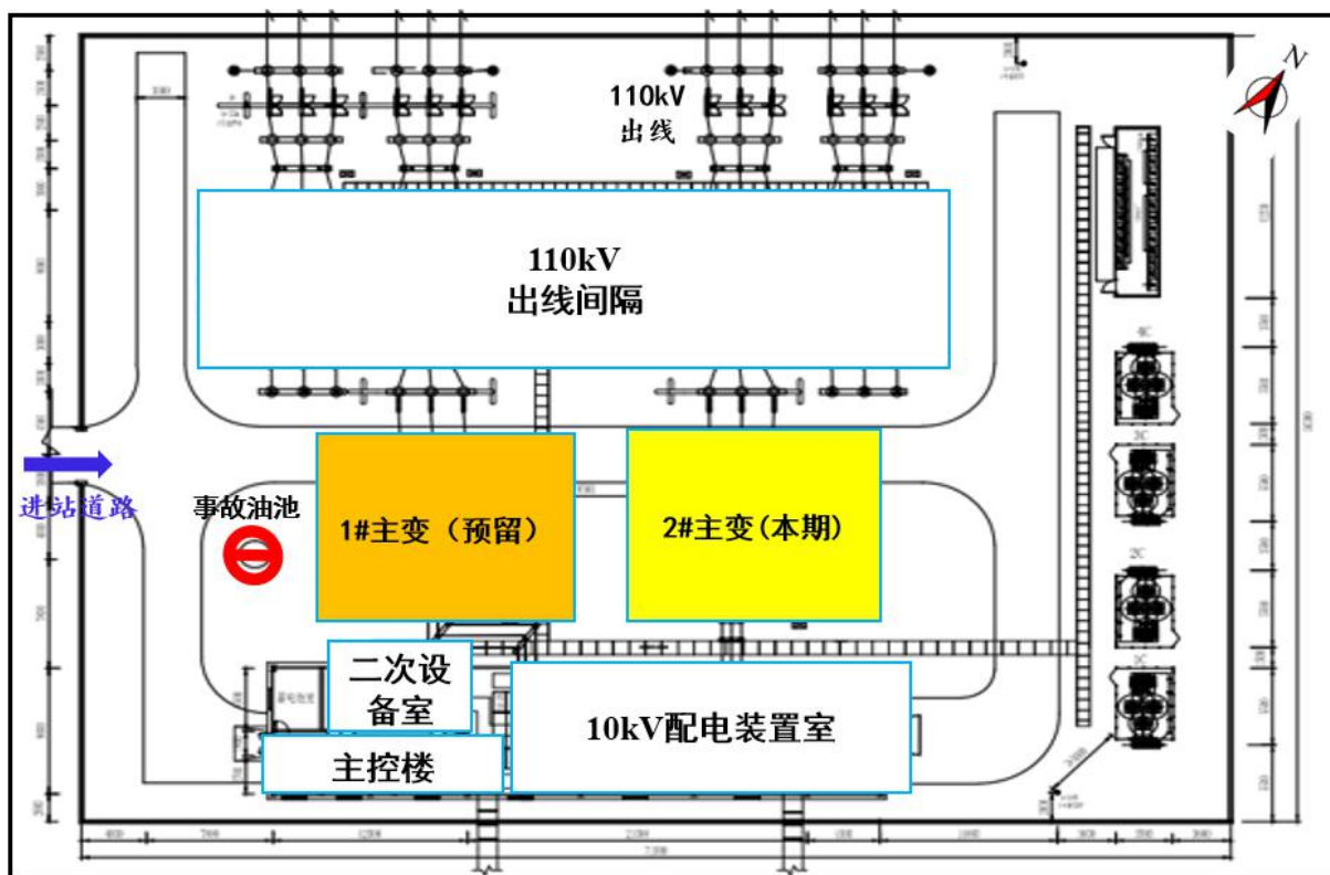
图 2 古家岭 110kV 变电站总平面布置示意
