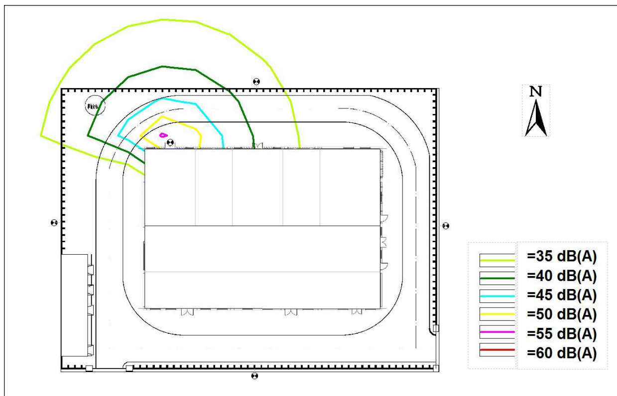
图 9 君山 110kV 变电站本期规模噪声预测等值线图
