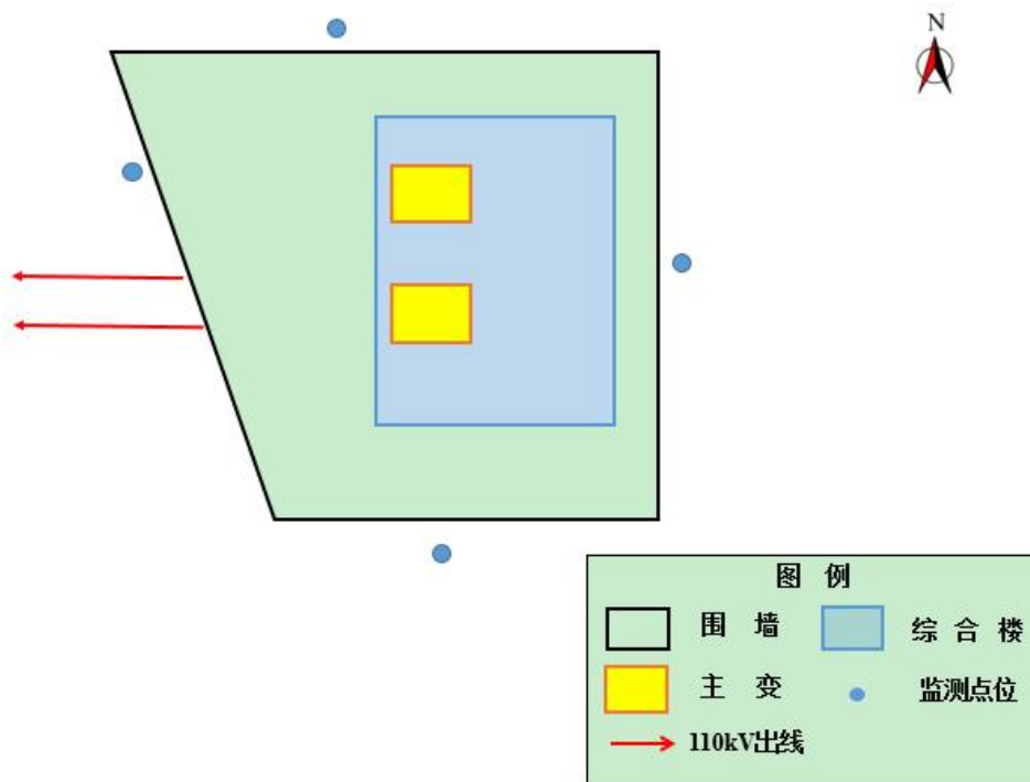
图 13 黑石铺 110kV 变电站平面布置及监测点位示意图
