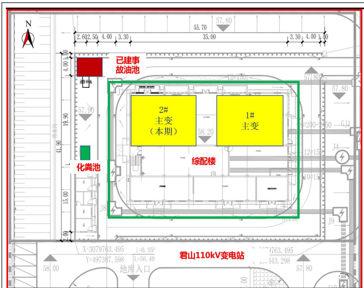
图 2 君山110kV变电站总平面布置图
