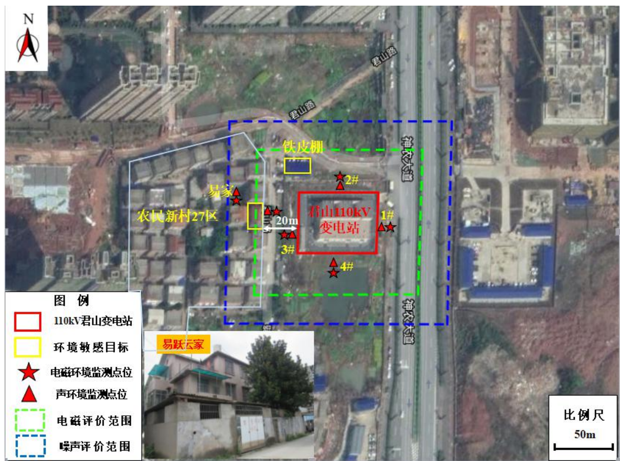
图 6 湖南株洲君山 110kV 变电站 2 号主变扩建工程与周边敏感点相对位置关系图
