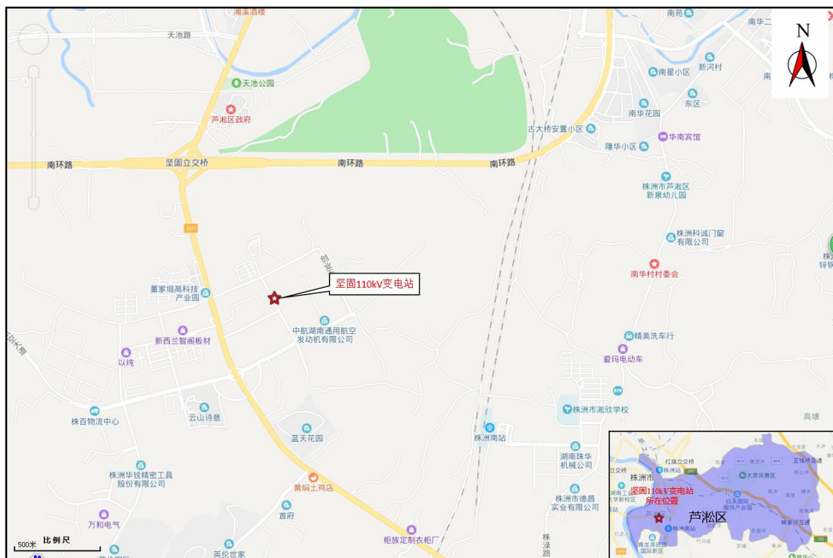
图 1 湖南株洲坚固110kV变电站2号主变扩建工程地理位置图
