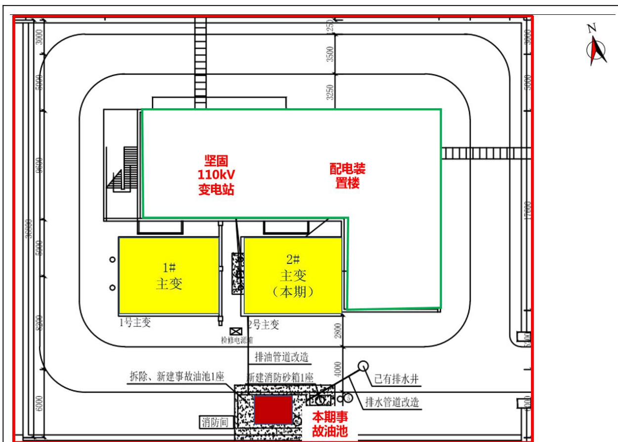
图 2 坚固110kV变电站总平面布置图
