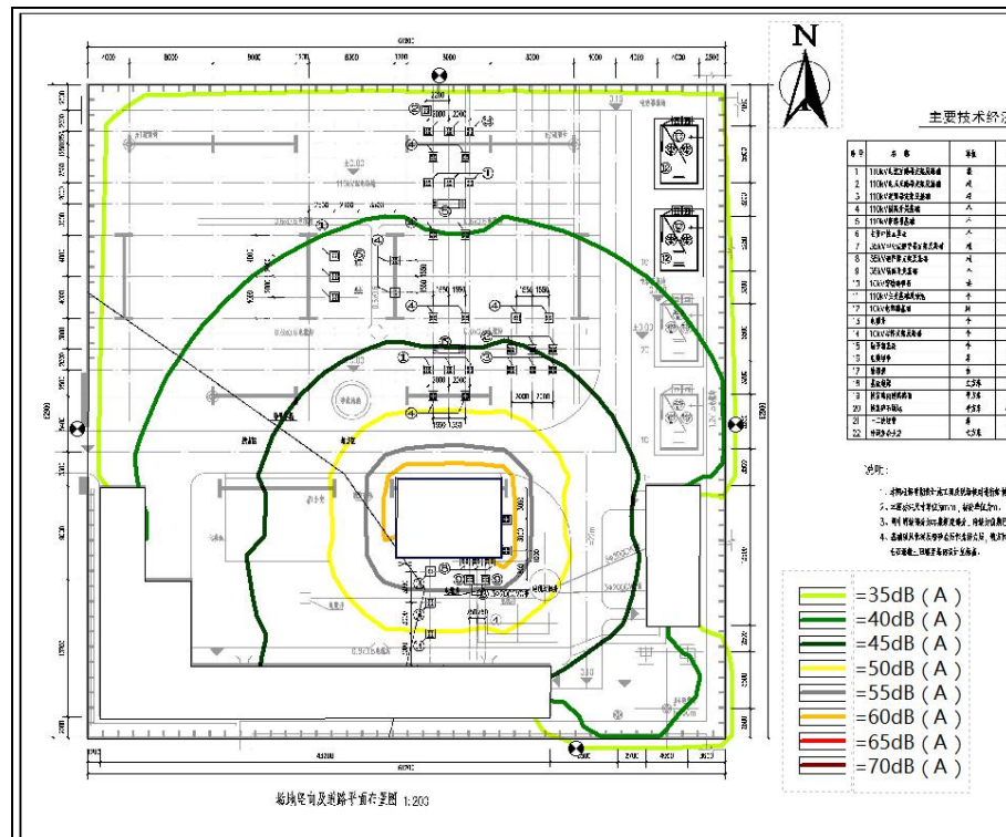
图 9 齐星 110kV 变电站本期规模噪声预测等值线图
