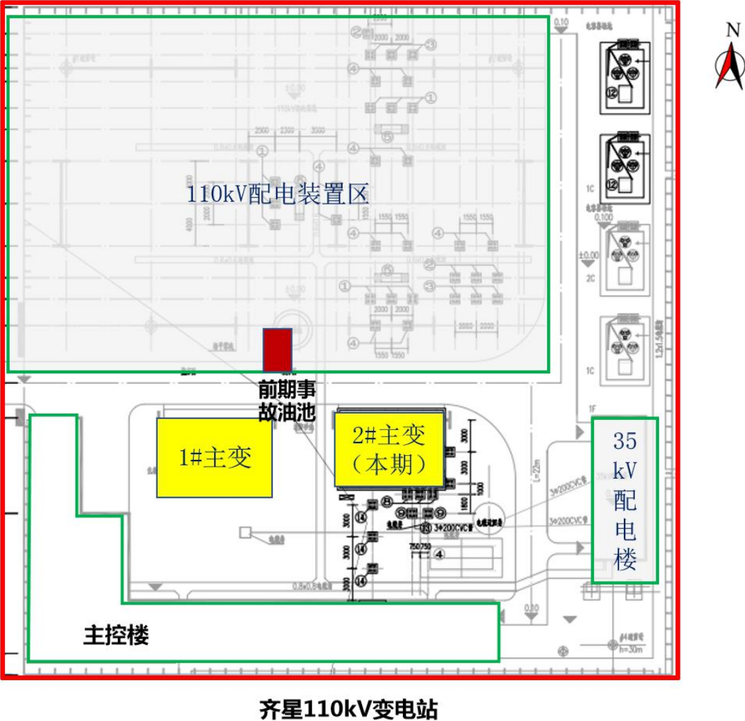
图 2 齐星 110kV 变电站总平面布置示意
