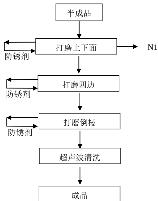
图 5 生产工艺流程及产污环节示意图
