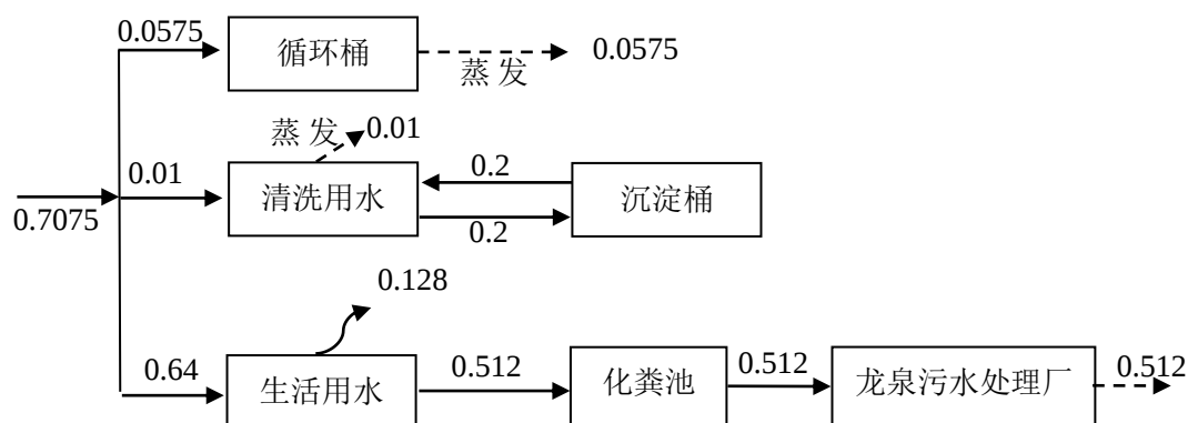
图 2 水平衡图 单位: \text{m}^3/\text{d}
